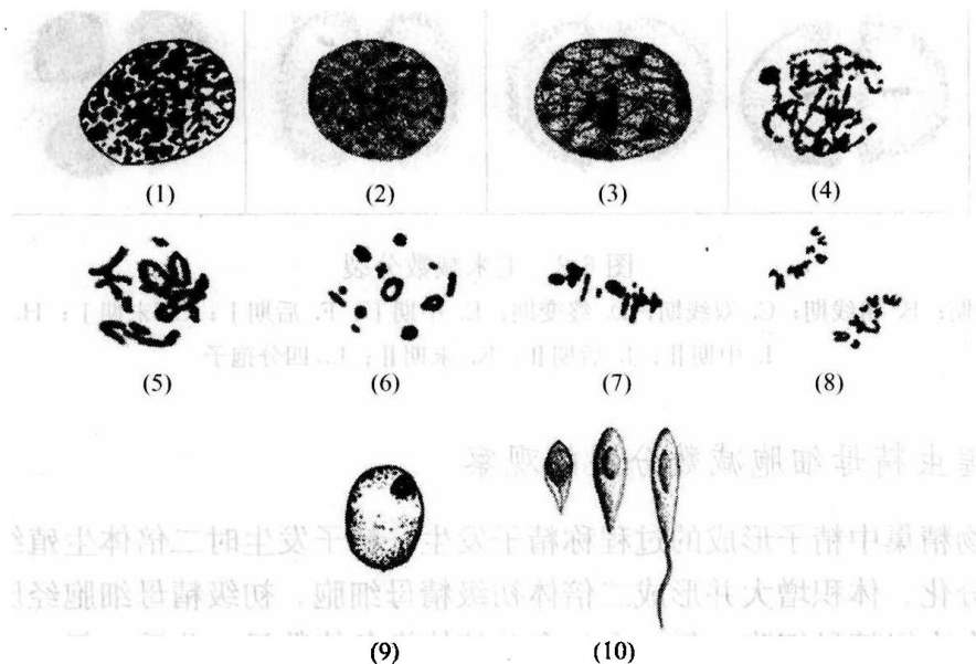
图 6-3 蝗虫精巢细胞减数分裂过程
