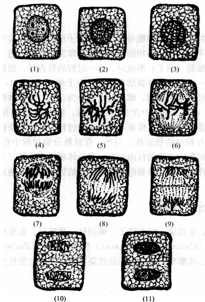
图 6-1 洋葱根尖细胞有丝分裂过程 (辛华, 2001)
