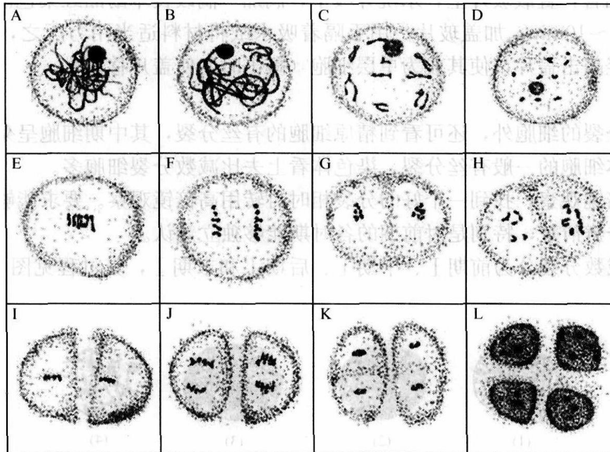
图 6-2 玉米减数分裂
