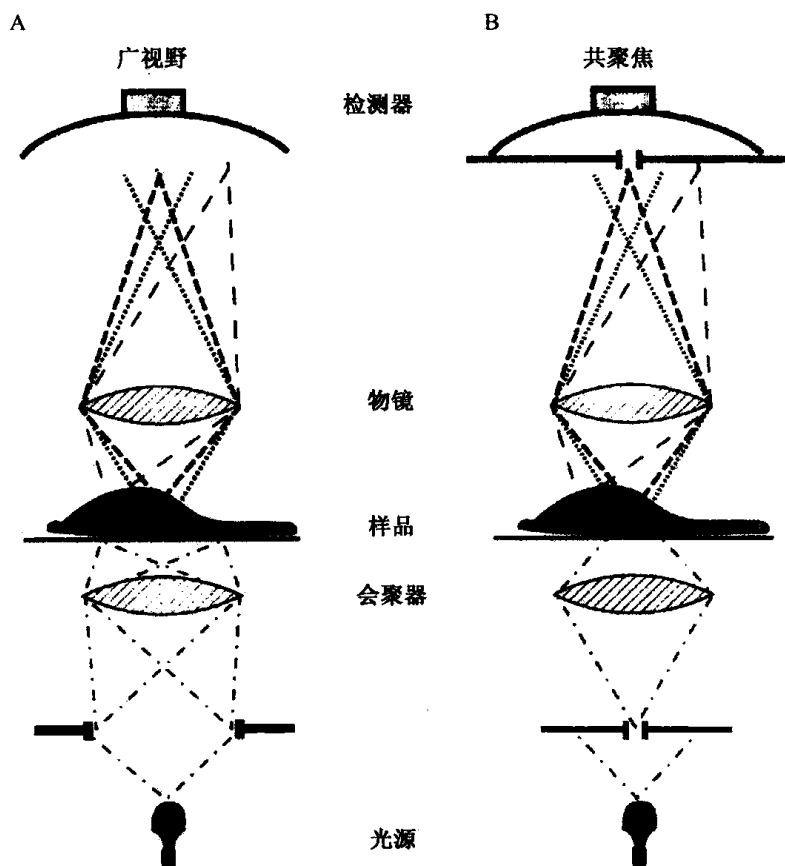
图 12-5 共聚焦显微镜操作原理示意图 (Spector et al., 1998)
