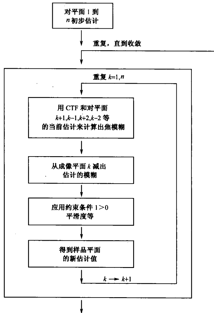
图 12-11 约束迭代去旋算法流程图 (Spector et al., 1998)
