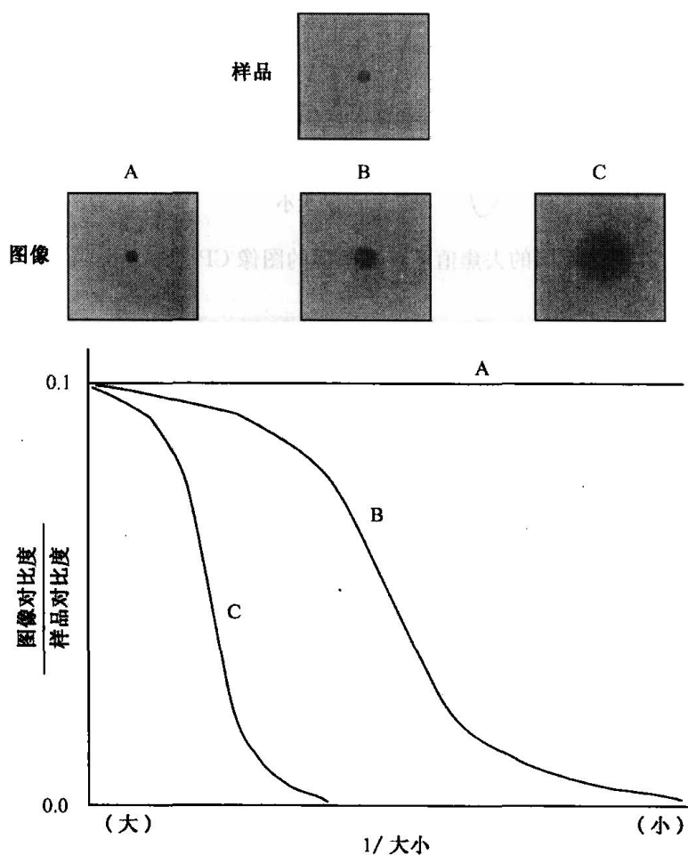
图 12-7 反差传递功能 (CTF) 示意图及相应的实物与成像效果对比图 (Spector et al., 1998)
