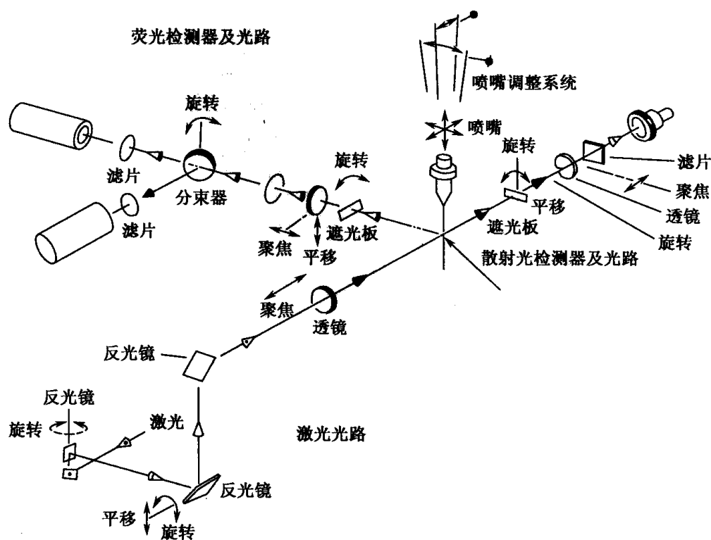
图 12-1 FACS440 光测量系统示意图 (刘鼎新和吕证宝, 1997)
