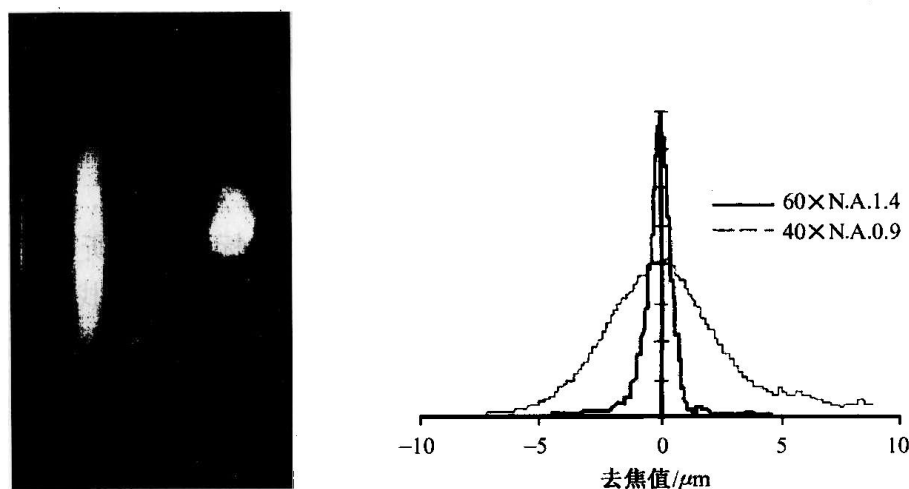
图 12-12 X-Z 扫描直径 0.9\mu\text{m} 的荧光珠并测量垂直点散功能 (Spector et al., 1998)
