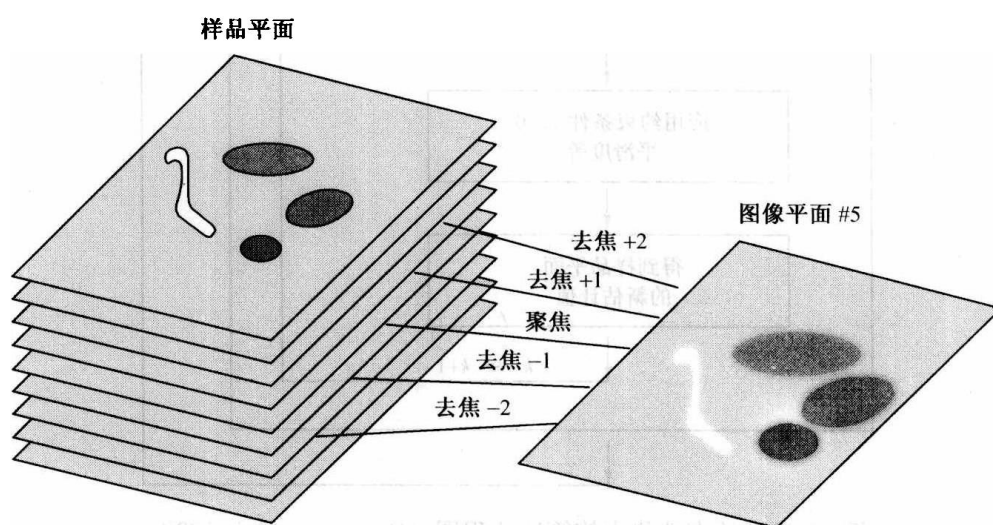
图 12-10 将一个聚焦平面图像加到在不同去焦程度下观察的邻近平面图上，形成厚样品图像 (Spector et al., 1998)
