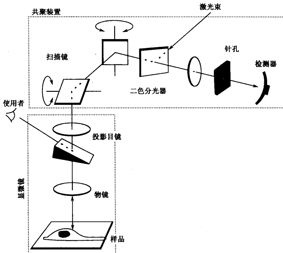
图 12-6 图中所画是一个典型的激光扫描共聚显微镜的构造图 (Spector et al., 1998) 仪器由一个荧光显微镜（在下方带阴影的长方形中）以及一个共焦扫描单元（上方带阴影的长方形所示）组成。共聚焦系统包括一对扫描镜、一束激光、一些波长选择滤片、一个针孔及一个光电倍增管检测器。照明激光被导向显微镜的光电管，经快速震荡的扫描镜改变方向以光栅的形式扫过样品，样品发出的荧光返回荧光管，被扫描镜“重新扫描”，经过二色分光器（可以去除所有反射的激光）到达针孔器。只有从焦平面发出的光经过针孔到达针孔器，其他光则被阻挡。对于反射成像，用半银镜代替二色分光器，通过移动一个棱镜片，使用者用普通的双目目镜，一般的照明光源，就可以转变成视野（共聚焦）观察
