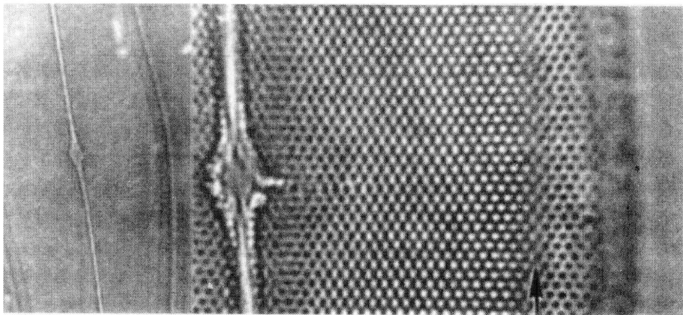
图 12-9 因去焦造成的对比度回复 (Spector et al., 1998)
