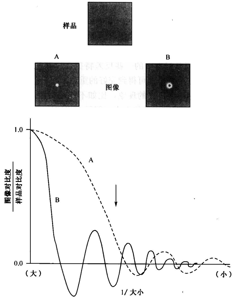
图 12-8 在两个不同的去焦值下，显微镜的图像 CP (Spector et al., 1998)
