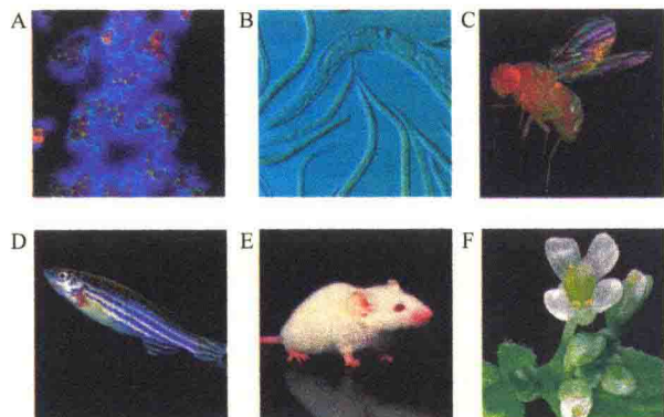
图 1-27 6 种真核生物研究的模式生物 (引自 Lodish et al., 2016)。A. 酵母, B. 线虫, C. 果蝇, D. 斑马鱼, E. 小鼠, F. 拟南芥。
