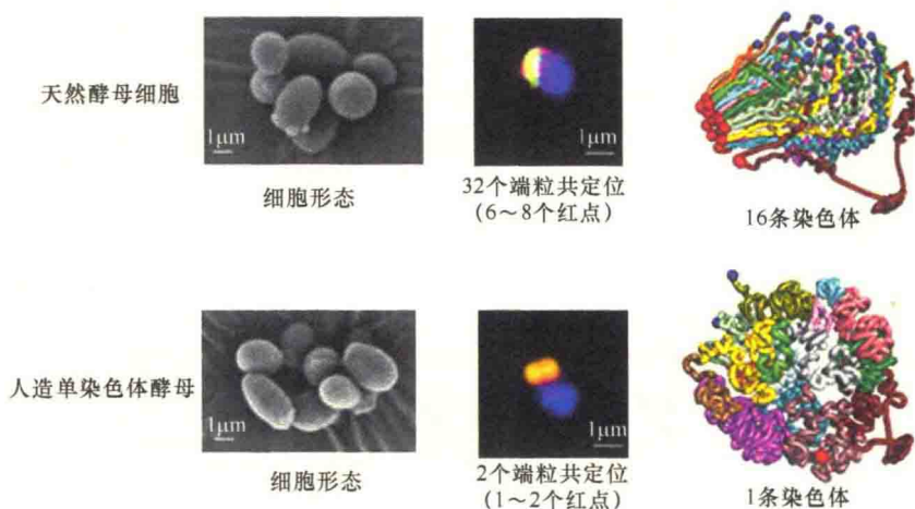
图 1-30 简约的 1 条染色体与 16 条染色体酵母的比较（引自 Shao et al., 2018）。
