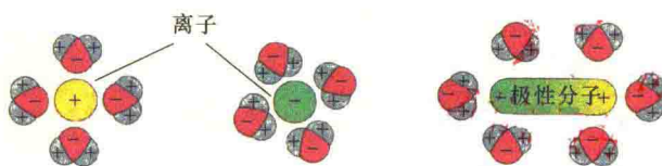
图 1-12 水的溶剂作用 (引自 Kleinsmith and Kish, 1995)。
