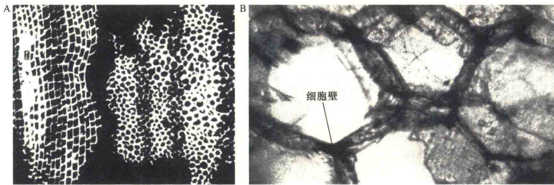
图 1-1 最早在显微镜下看到的细胞结构（引自 Kleinsmith and Kish, 1995）。A. 1665 年胡克论文中展示的栎树细胞，仅是植物组织死细胞的细胞壁；B. 1674 年列文虎克观察到的细胞结构，其细胞壁的结构十分明显，但是看不到细胞内的结构。
