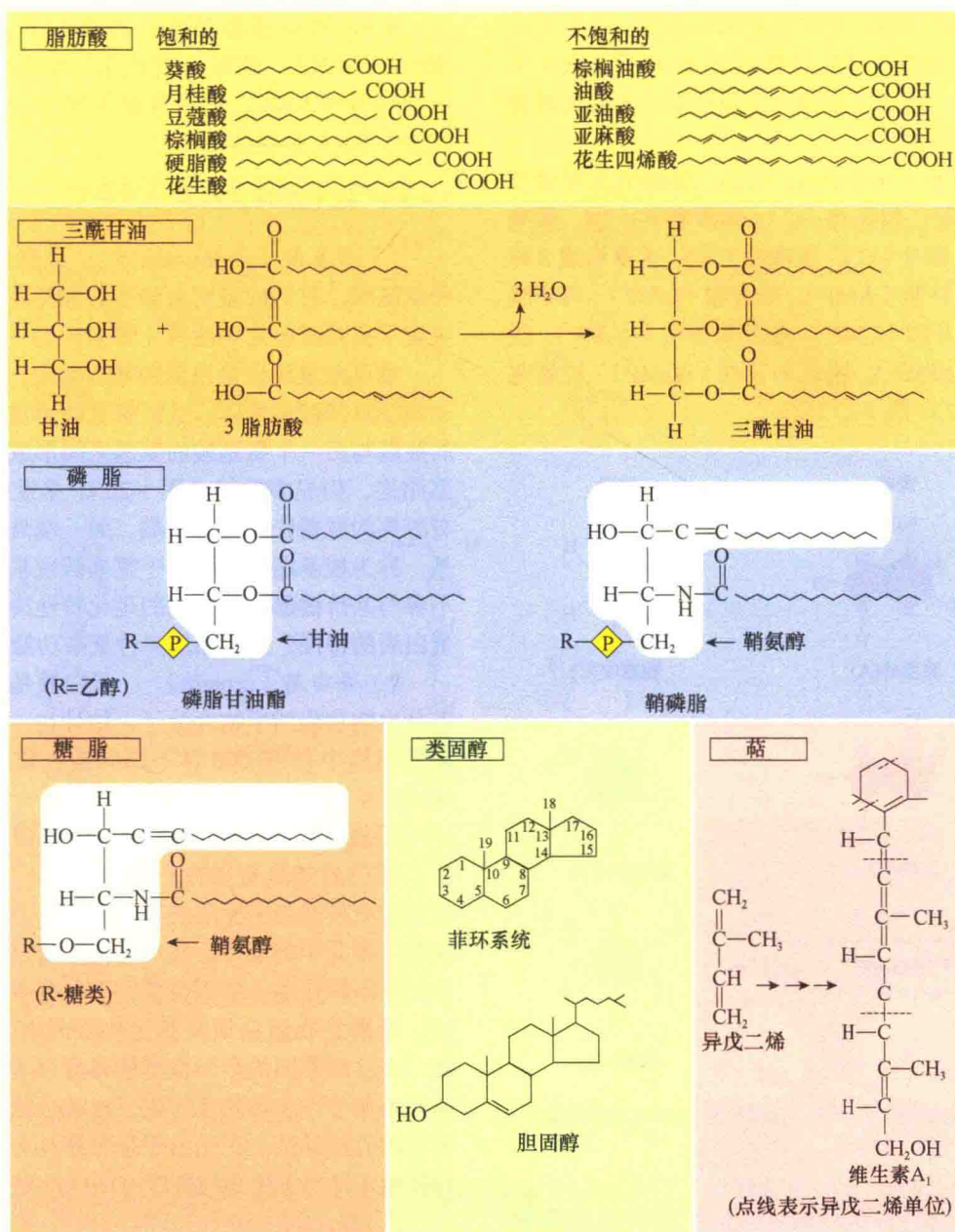
图 1-15 细胞内 6 类不同的脂 (引自 Kleinsmith and Kish, 1995)。
