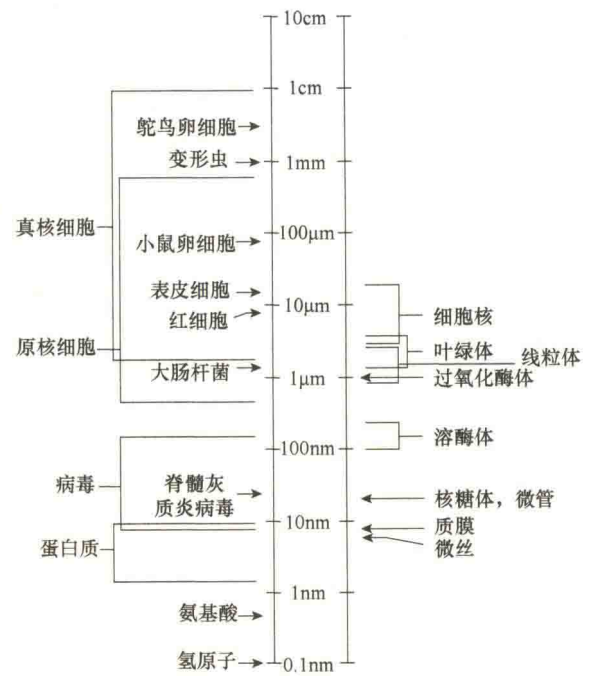
图 1-7 典型的原核细胞、真核细胞、细胞器、病毒和分子的大小（引自 Kleinsmith and Kish, 1995）。
