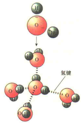
图 1-11 水分子中的氢键（引自 Kleinsmith and Kish, 1995）。
