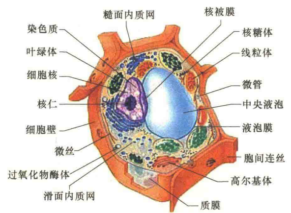
图 1-5 植物细胞模式图。
