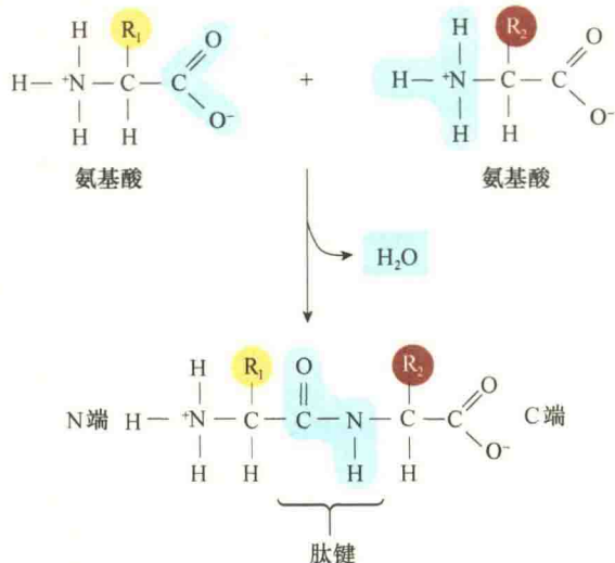
图 1-20 两个氨基酸之间通过脱水形成肽键。
