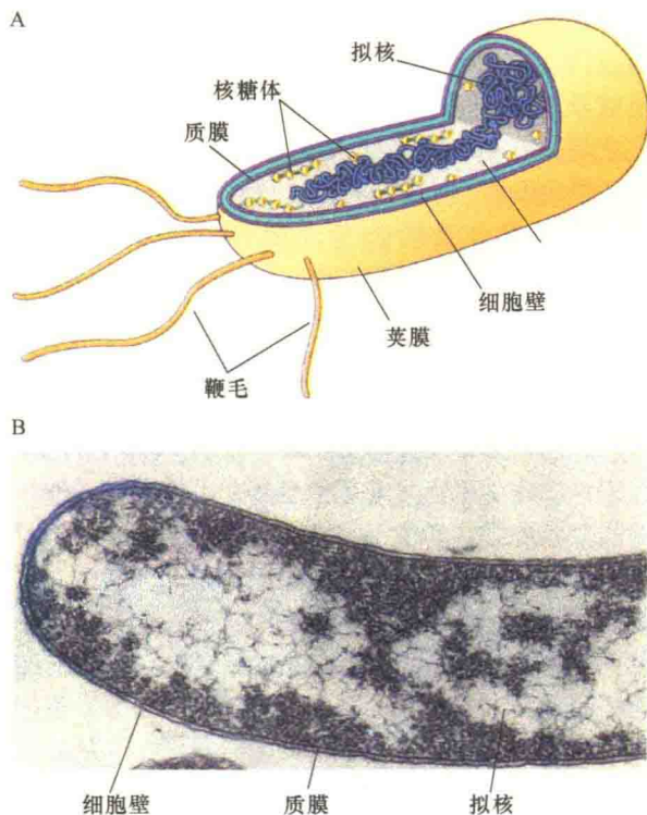
图 1-2 典型细菌细胞形态结构 (引自 Kleinsmith and Kish, 1995)。A. 细菌的三维结构。B. 革兰氏阳性菌切片的电子显微镜照片。
