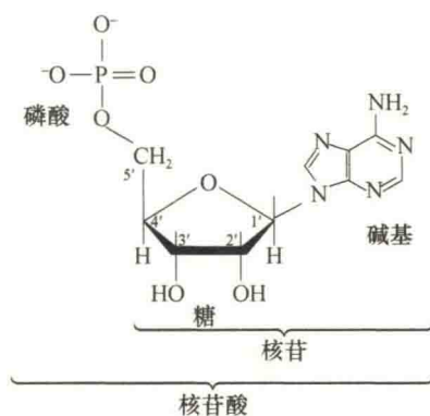
图 1-16 核苷酸的组成单位 (引自 Kleinsmith and Kish, 1995)。
