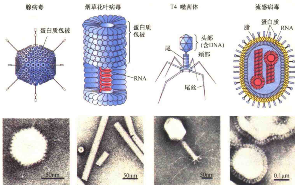
图 1-22 常见病毒的形态和结构 (引自 Kleinsmith and Kish, 1995)。上面一行是结构模式图, 下面一行是电子显微镜照片。
