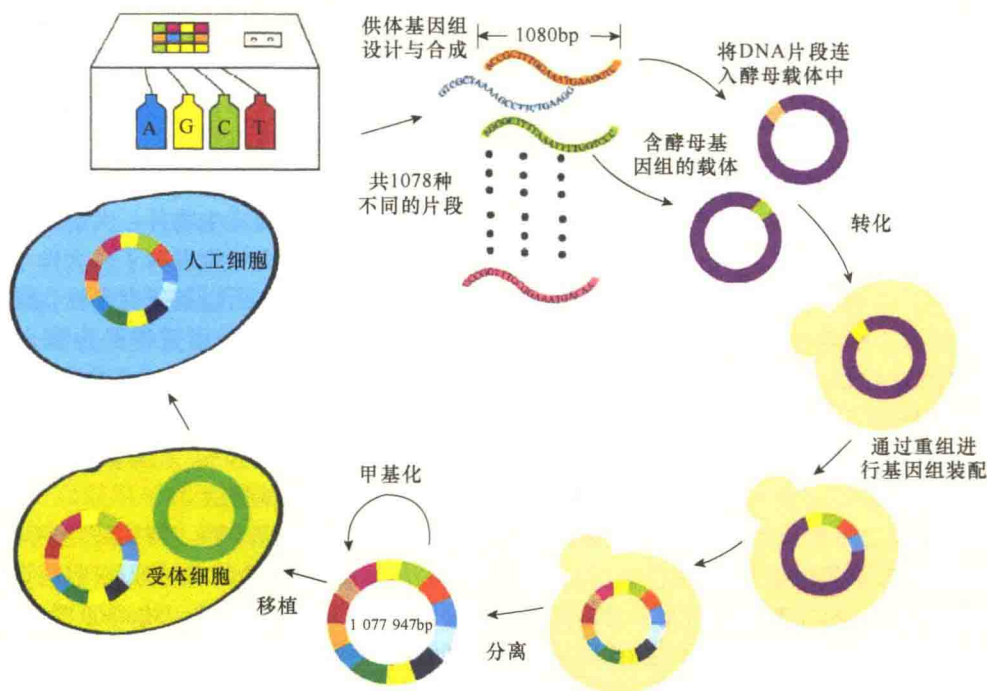
图 1-29 “Synthia”的诞生过程(引自孙明伟等, 2010)。
