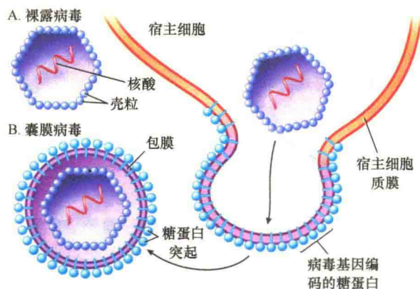
图 1-23 囊膜病毒的形成 (引自 Solomon et al., 2019)。
