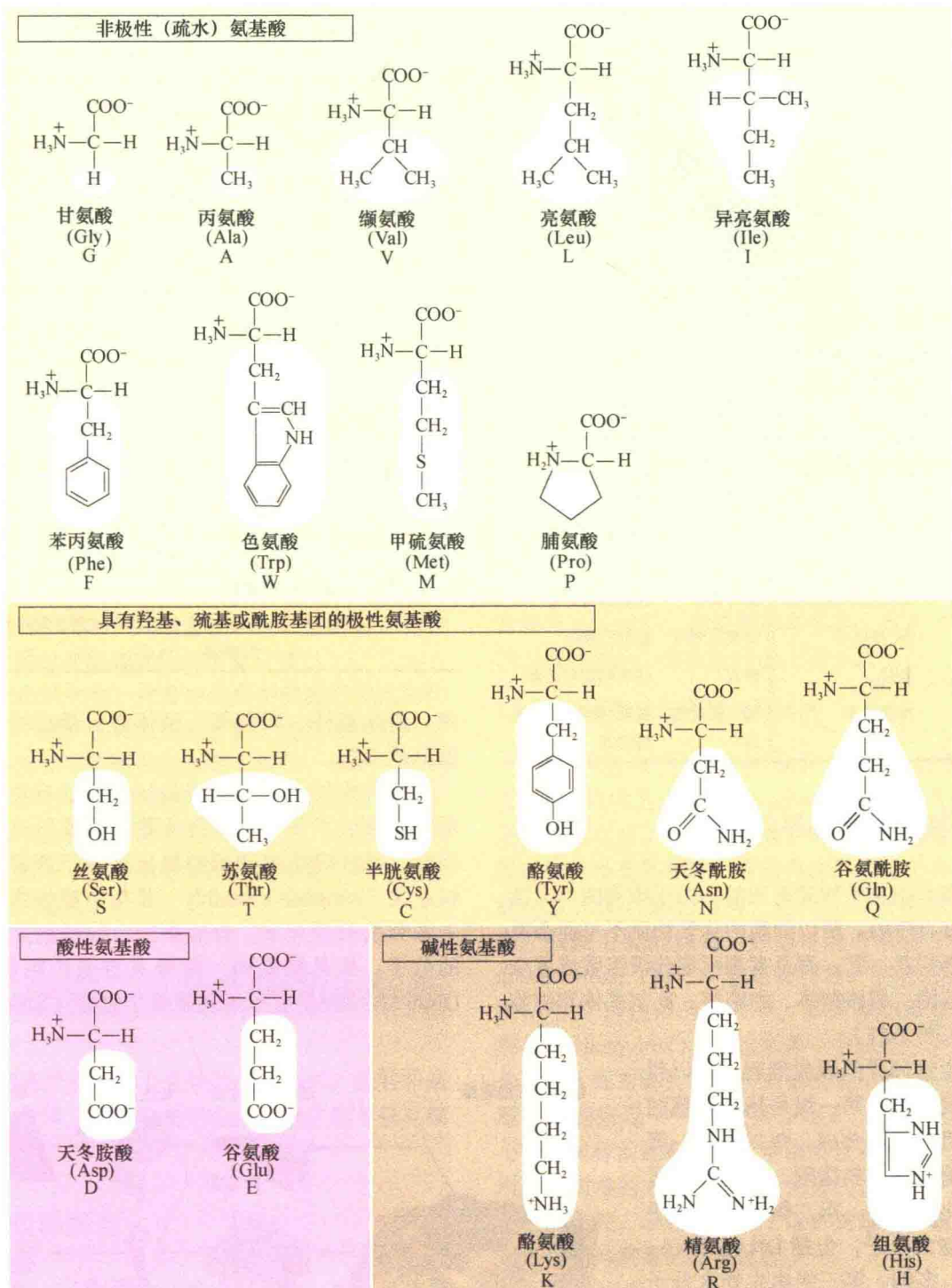
图 1-19 20 种氨基酸的结构。
