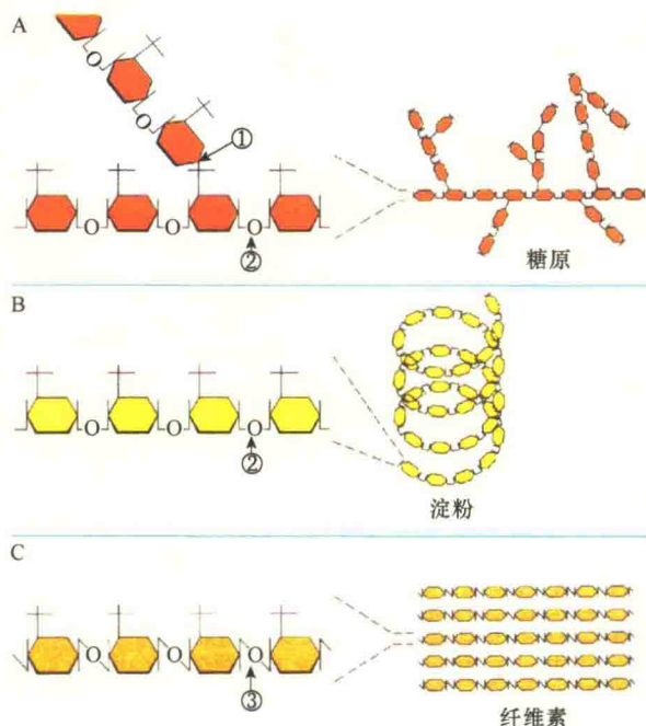
图 1-14 相同的单糖构成不同的多糖 (引自 Karp, 1996)。圆圈数字箭头表示三种不同的连接方式。
