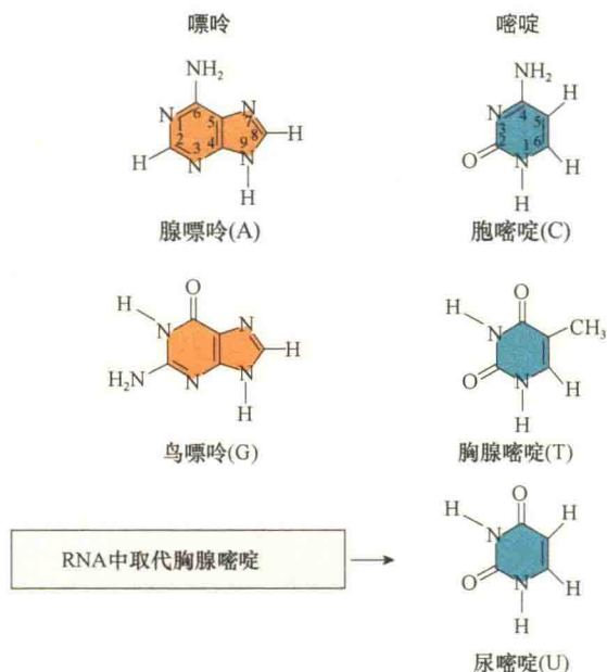
图 1-17 核苷酸中的碱基 (引自 Kleinsmith and Kish, 1995)。
