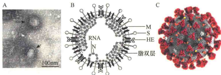
图 1-24 冠状病毒的形态结构。A. 中国国家病原微生物资源库发布的 SARS-CoV-2 病毒的电镜照片 (箭头处)。B. 冠状病毒包膜及突起蛋白。图中 N 表示核衣壳蛋白。C. 冠状病毒的形态。
