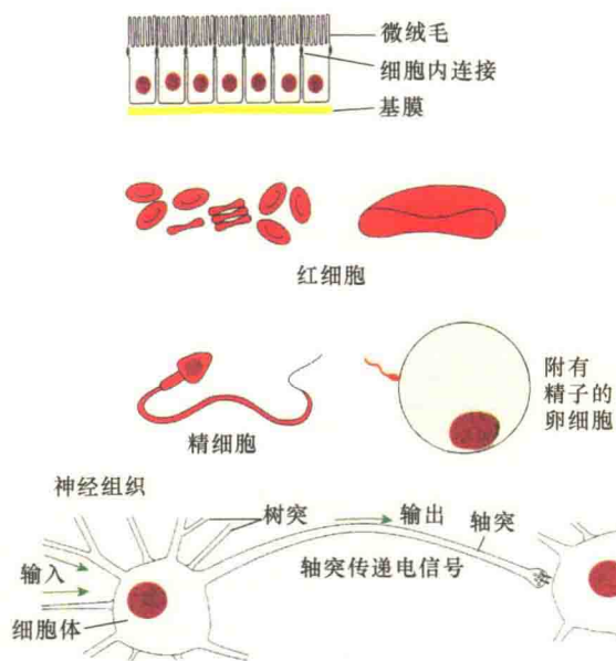
图 1-6 不同的细胞形态 (改编自 Alberts et al., 1994)。
