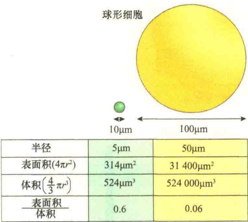
图 1-8 细胞体积与表面积间的关系（引自 Kleinsmith and Kish, 1995）。
