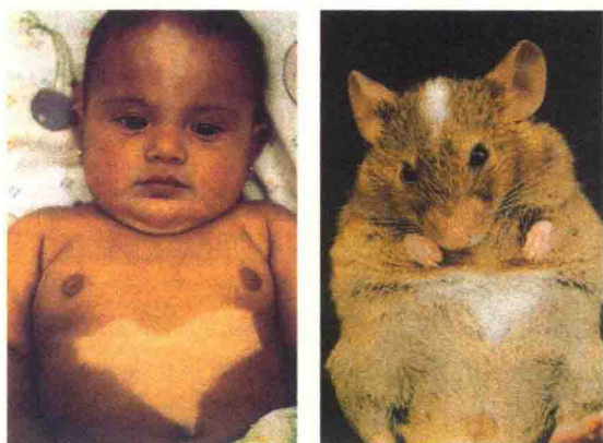
图 1-28 小鼠作为研究人的发育模式生物(引自 Cooper and Hausman, 2013)。一个小孩与一只小鼠同一个基因突变造成相同的遗传缺陷。图示胸前的白斑是因为一个基因的突变影响了胚胎发育期黑素细胞的正常迁移所致。
