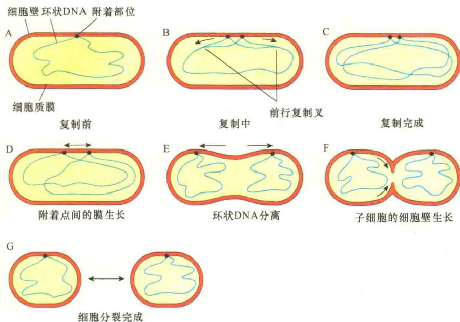
图 1-3 细菌的细胞质膜参与环状 DNA 的复制与分裂 (引自 Wolfe, 1993)。
