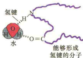
图 1-12 水的溶剂作用 (引自 Kleinsmith and Kish, 1995)。
