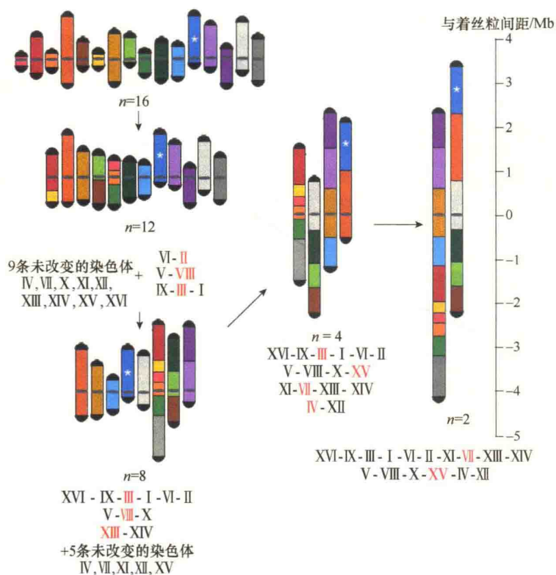
图 1-31 简约的 2 条染色体的策略 (引自 Luo et al., 2018)。
