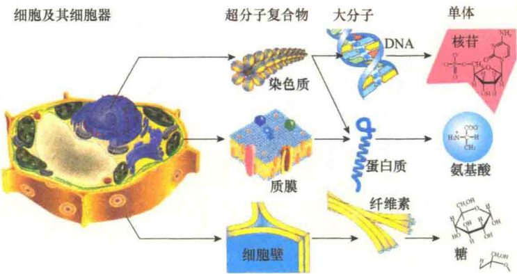
图 1-21 植物细胞的化学组装（引自 Nelson and Cox，2013）。
