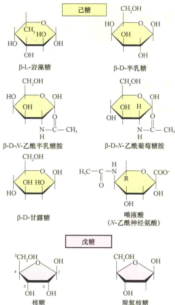
图 1-13 一些重要的单糖 (引自 Kleinsmith and Kish, 1995)。
