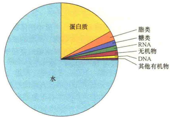
图 1-10 细胞中各主要成分的相对含量（引自 Kleinsmith and Kish, 1995）。
