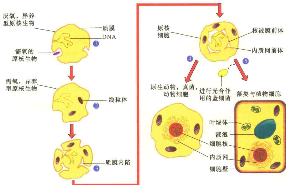
图 1-26 真核细胞的进化 (引自 Karp, 2010)。进化分为 5 个过程: ①一个大的厌氧菌——异养菌吸收了一个小的需氧原核生物, 有研究证明所吞的细菌是现今自然界存在的立克次氏体的祖先; ②被吞入的好氧细菌进化成线粒体; ③部分细胞质膜内陷, 形成核膜、内质网膜的前体, 形成初级真核细胞; ④初级真核细胞继续进化成为无光合作用的原生动物、动物细胞; ⑤在另一个途径, 初级真核细胞吞入了具有光合作用的细菌, 该细菌逐渐内化并演化成植物细胞的叶绿体。
