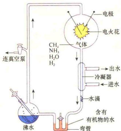
图 1-25 Miller 推测地球上的有机分子自动合成的实验装置(引自 Wolfe, 1993)。
