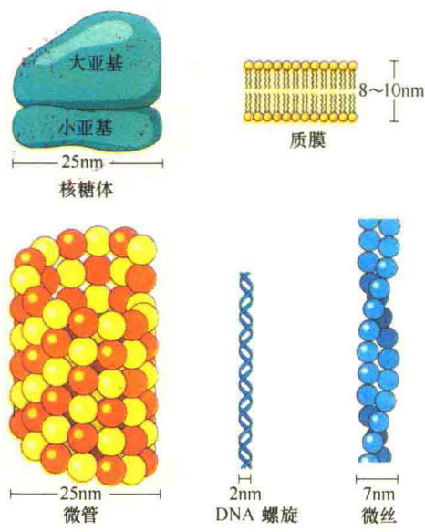
图 1-9 几种细胞结构的大小（引自 Becker et al., 1996）。
