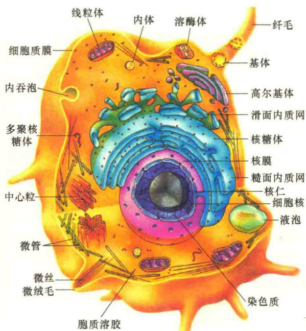
图 1-4 动物细胞模式图。
