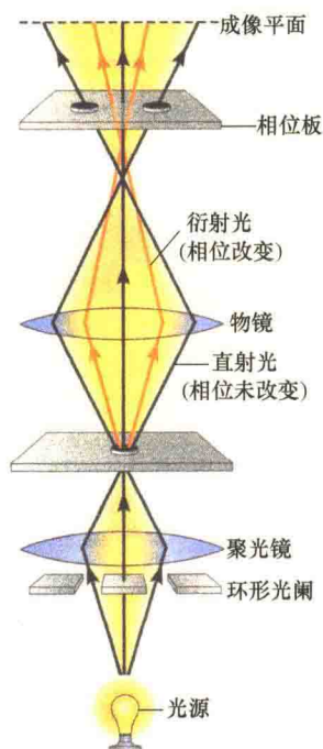
图 2-8 相差显微镜的光学组件及光线通路（引自 Jeff et al., 2012）。橙色线代表由标本干涉的光，黑色线代表直射光。
