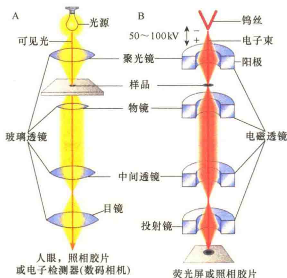
图 2-1 光学显微镜与电子显微镜的光学系统(引自 Hardin et al., 2012)。A. 光学显微镜用可见光(波长 400\sim 700\text{nm} )与玻璃透镜将标本转变成肉眼、胶片或数码相机接收的影像。B. 电子显微镜利用钨丝发射的电子束,通过电磁透镜聚焦将标本在荧光屏、数字检测器及胶片上成像。
