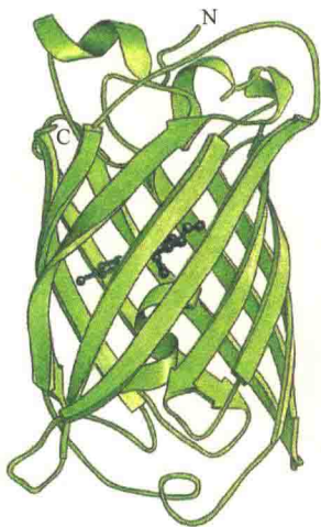
图 2-19 绿色荧光蛋白（GFP）的结构（引自 Alberts et al., 2015）。GFP 由 13 条 β 链形成一个桶状结构，活性的发色团包含在桶的内部，它是翻译后由三个氨基酸残基伸出的侧链。
