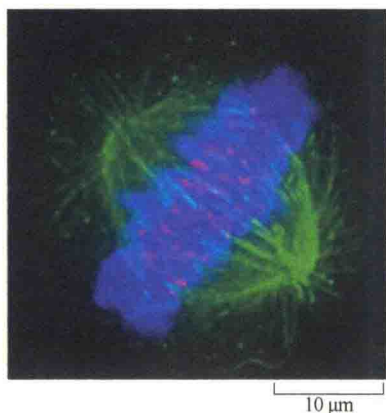
图 2-17 同一个细胞可同时用不同的探针进行观察(引自 Alberts et al., 2015)。照片显示了细胞有丝分裂的纺锤体及染色体。用三种不同的荧光探针标记三种不同的细胞组分: 纺锤体微管用绿色荧光抗体进行标记, 着丝粒用红色荧光抗体进行标记, 凝聚染色体的 DNA 用蓝色荧光染料 DAPI (可与 DNA 沟结合的染料) 标记。
