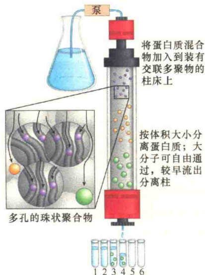
图 2-39 根据分子大小分离蛋白质的凝胶过滤层析法 (引自 Nelson and Cox, 2013)。将蛋白质混合液从顶部泵入用多孔的聚合物凝胶小球填充的层析柱, 小蛋白质通过柱床时经由凝胶珠子的孔进入凝胶, 而大的蛋白质则不会进入凝胶珠子, 速度不会受阻, 所以小蛋白质的速度要比大蛋白质的流动速度慢, 因此, 不同大小的蛋白质被洗脱出层析柱的时间也就不同, 可被分部分 (fraction) 收集到不同的蛋白收集管中。
