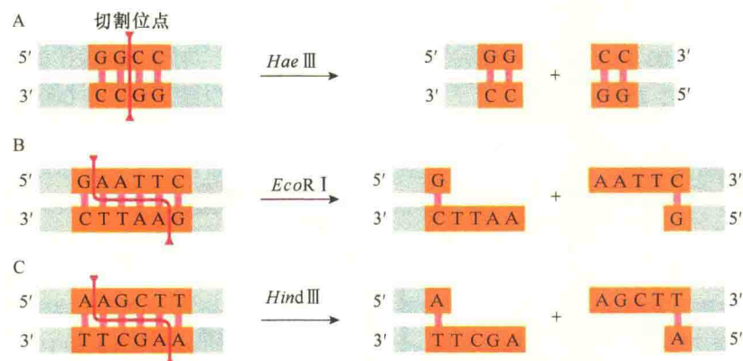
图 2-46 限制性内切核酸酶切割产生的黏性末端与平末端 (引自 Alberts et al., 2015)。A. 限制性内切核酸酶 Hae III 识别靶序列后在两条链中轴线切割, 产生具有平末端的产物; B. 限制性内切核酸酶 Eco R I 识别序列后, 在两条链的识别序列的交错部位切割, 产生具有 5' 端的产物; C. 限制性内切核酸酶 Hind III 识别序列后, 在两条链的识别序列的交错部位切割, 产生具有 5' 端的产物。
