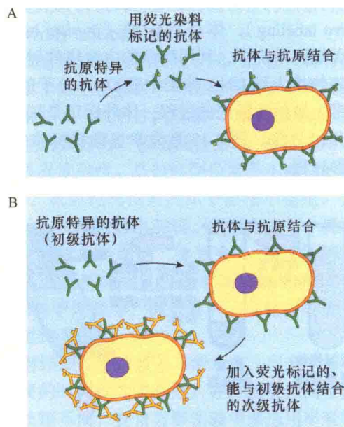
图 2-16 用荧光抗体进行免疫染色 (引自 Jeff et al., 2012)。免疫荧光显微镜用荧光标记的抗体检测组织样品中特异的分子(抗原)。A. 直接免疫荧光。使用的与组织内特异分子结合的抗体是用荧光染料标记的,将这种标记的抗体加入到样品中,使之与检测的抗原结合,然后用荧光显微镜或共聚焦显微镜进行检测。B. 间接免疫荧光。使用两种抗体,初级抗体不用标记,并且直接与待检测的特异抗原结合。随后加入的次级抗体是用荧光标记的,但并不与待检测的抗原结合,而是与未标记的初级抗体结合,间接免疫荧光有效扩增了荧光信号,检测样品敏感性比直接荧光高得多。
