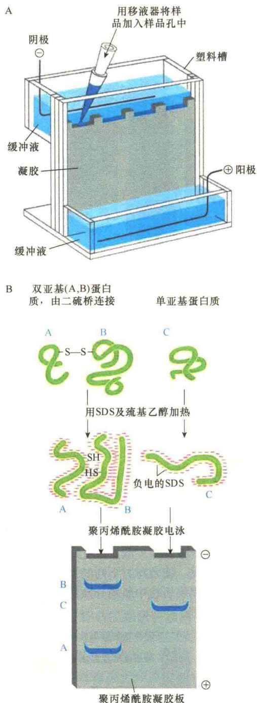
图 2-42 SDS-聚丙烯酰胺凝胶电泳 (引自 Alberts et al., 2015)。A. 电泳装置; B. 以三种蛋白质单体显示分离的原理及最后形成的蛋白质带形。
