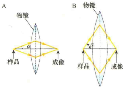
图 2-4 透镜的角孔径（引自 Becker et al., 1996）。角孔径是光从标本进入透镜的半角（ \alpha ）。A. 小孔径透镜；B. 大孔径透镜。角孔径越大，透过透镜的信息越多。
