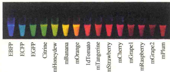
图 2-20 多种不同颜色的荧光蛋白（引自 Lodish et al., 2013）。图示发射不同荧光的试管及所含荧光蛋白的名称。
