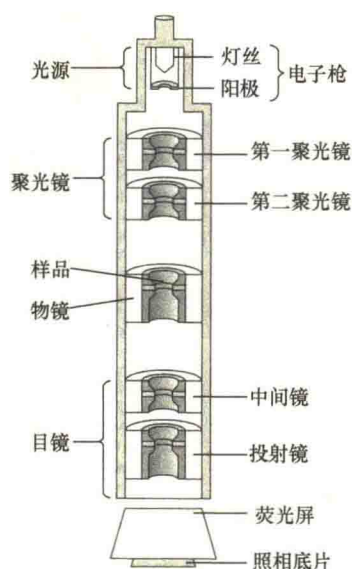
图 2-24 透射电子显微镜的电子光学系统 (引自 Wolfe, 1993)。
