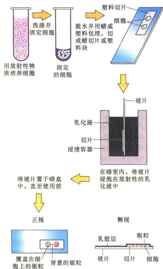
图 2-13 光学显微镜标本的放射自显影（引自 Karp, 2010）。
