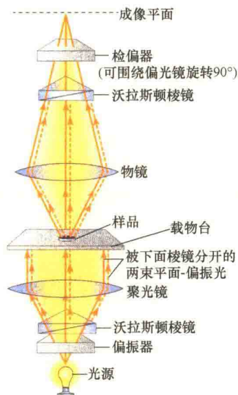
图 2-9 微分干涉相差（DIC）显微镜的光学组件及光线通路（引自 Jeff et al., 2012）。
