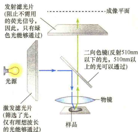
图 2-15 荧光显微镜的基本结构与光通路 (引自 Jeff et al., 2012)。光源发射的荧光通过激发滤光片的阻断作用,仅让激发光通过(蓝色线条),激发光诱发样品中的荧光染料发射较长波长的光(绿色线条),发射滤光片除去激发光,仅允许发射光通过,最后,样品中荧光分子发射的光形成影像。
