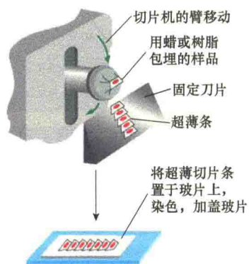
图 2-12 用切片机进行标本切片（引自 Jeff et al., 2012）。将固定的标本包埋之后，固定在切片机的臂上，当切片机的臂通过一个环形的弧光刀，就会将标本切成切片。这些切片互相粘在一起，形成橡皮条状，然后可以固定在玻片上，进行染色并加上盖玻片保护起来。
