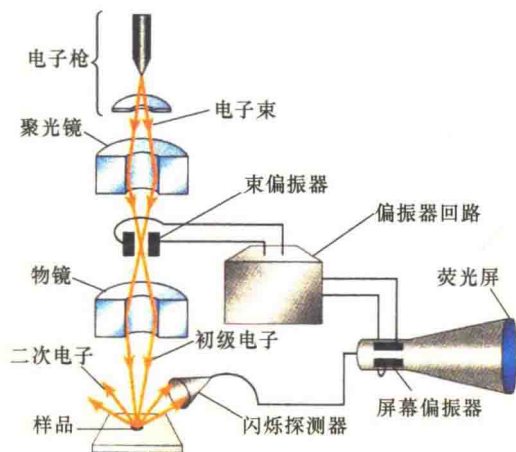
图 2-25 扫描电子显微镜的光学系统（引自 Jeff et al., 2012）。
