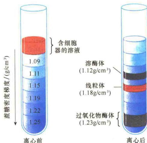
图 2-35 密度梯度离心分离溶酶体、线粒体和过氧化物酶体(引自 Lodish et al., 2013)。
