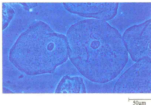
图 2-7 相差显微镜观察的上皮细胞显微照片 (引自 Becker et al., 1996)。上皮细胞未经处理及染色, 直接在相差显微镜下进行观察。
