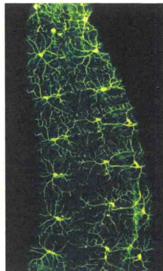
图 2-21 荧光蛋白作为报告蛋白（引自 Alberts et al., 2015）。通过 DNA 重组技术，将 GFP 编码序列置于果蝇的启动子控制下，该启动子只能在一套特异的神经元中被激活。图中的影像是通过荧光显微镜拍摄的活果蝇胚，显示了约 20 个神经元，每个神经元具有很多轴突和树突，与周围非荧光的细胞进行通讯。这些神经元刚好位于动物的表面，可敏感地感知环境。
