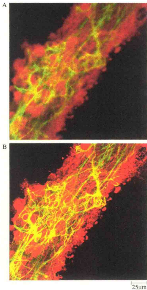
图 2-18 共聚焦荧光显微镜与普通荧光显微镜的比较 (引自 Jeff et al., 2012)。图中的荧光照片显示的是用不同的荧光标记物染色的、用荧光标记的胶质细胞 (红色)、神经细胞 (绿色)。A. 一般的荧光显微镜照片, 整个样品都是被光照的, 所以在聚焦的平面、上方、下方的荧光材料都会形成模糊的影像。B. 在共聚焦显微镜中, 进入的光被聚焦在单个的平面, 从样品发射的焦外荧光则被排除了, 产生的影像泾渭分明。
