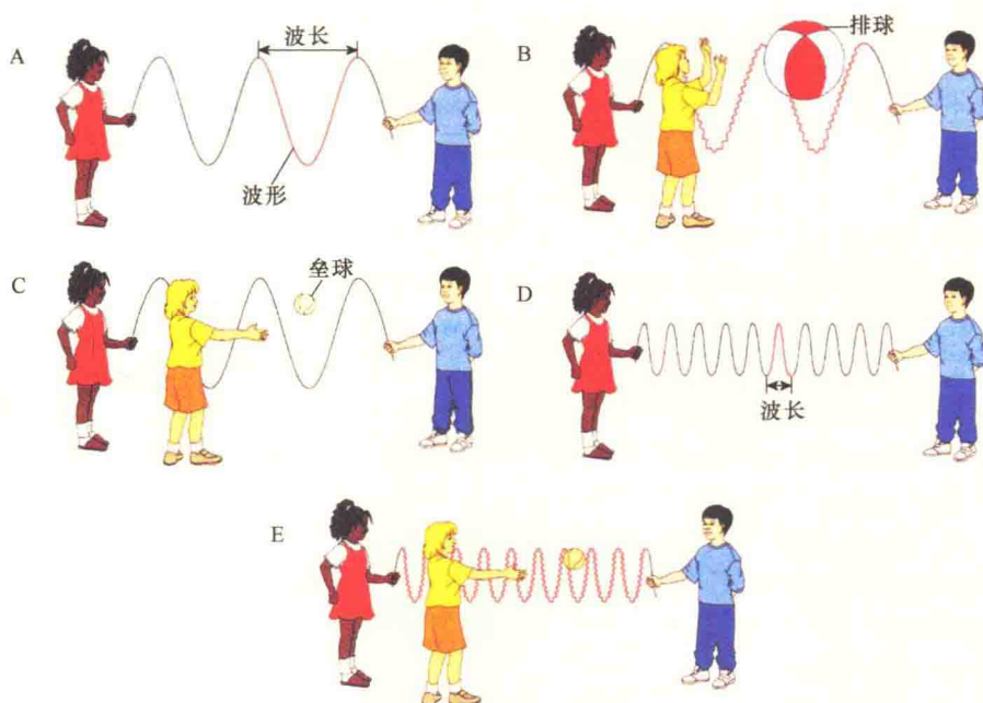
图 2-2 波的移动、波长与干扰(引自 Becker et al., 1996)。两个儿童共同振动一条绳子产生的波形类似于光子和电子形成的波动,以此说明物体的大小对波的干扰。A. 两个儿童振动绳子产生的特征波长;B. 向绳子波中扔进一个排球或一个物体,如果扔进物体的直径与绳子波长相近,就会干扰绳子波的移动;C. 如果扔进一个垒球或其他比绳子波长小得多的物体,对绳子波的移动只有很小或没有干扰;D. 如果将绳子快速振动,波长就会大大缩短;E. 此时扔进垒球就会干扰绳子波的移动。
