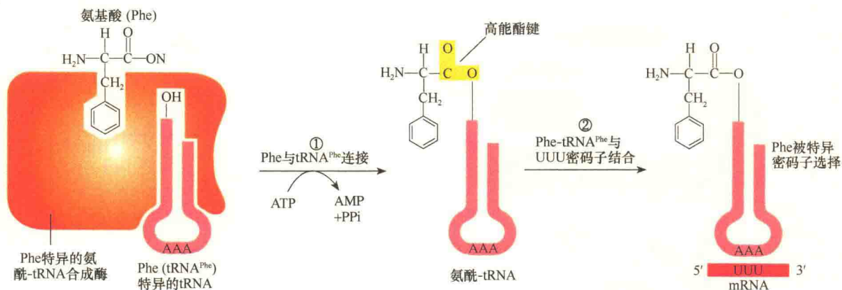
图 6-16 将核酸序列解码成氨基酸序列（引自 Lodish et al., 2013）。在蛋白质合成中，将 mRNA 中的核酸序列翻译成氨基酸序列，涉及两个步骤：①氨酰 tRNA 合成酶先与特异的氨基酸偶联，经由一个高能酯键与相应 tRNA 末端的腺嘌呤 2' 或 3' 羟基相连；②氨酰 tRNA 反密码环中的 3 个碱基序列通过配对规律与 mRNA 中对应的密码子序列配对，从而对 mRNA 中的密码子进行解码。
