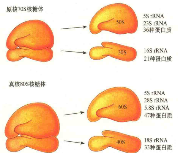
图 6-1 核糖体的结构（引自 Cooper and Hausman, 2013）。
