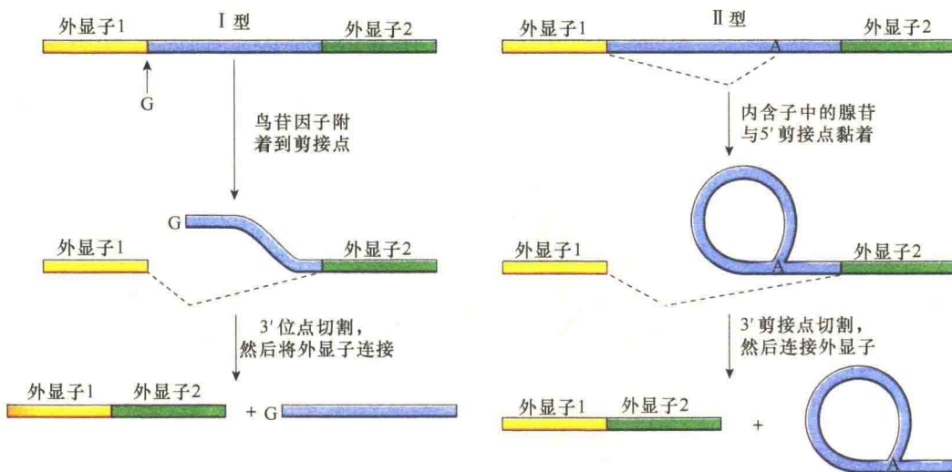
图 6-36 I 型内含子、II 型内含子自我剪接 (引自 Cooper et al., 2013)。在 I 型内含子剪接中, 剪接反应的第一步, 在鸟苷 (G) 的引导下, 在内含子的 5' 端剪接点进行切割, 生成一种线性的、内含子 5' 端结合有 G 的中间体。在 II 型内含子的剪接中, 剪接反应的第一步是通过内含子内的腺苷反应进行 5' 剪接点切割, 形成套索中间体。I 型内含子和 II 型内含子剪接的第二步都是在 3' 端剪接点进行切割, 然后进行外显子的连接。
