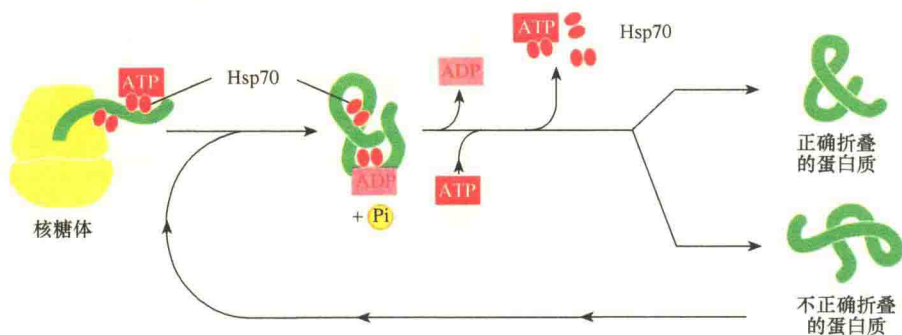
图 6-24 分子伴侣 Hsp70 家族介导的蛋白质折叠（引自 Alberts et al., 2015）。这类分子伴侣工作较早，核糖体上合成的新生肽露出一小段就被 Hsp70 分子伴侣所识别并与之结合，在一组小分子 Hsp40（未显示）的协同下，ATP 与 Hsp70 结合，然后将 ATP 水解成 ADP，帮助靶蛋白折叠后离开。若是折叠不正确，重新进行折叠。
