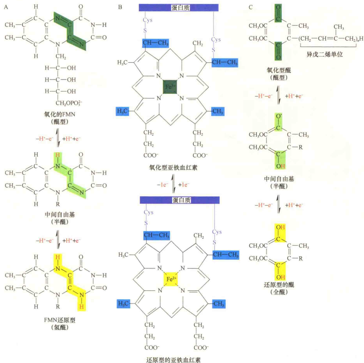
图 7-14 三种电子载体的氧化与还原结构 (引自 Karp, 2010)。A. NADH 脱氢酶的 FMN (黄素单核苷酸); B. 细胞色素 c 的血红素基团; C. 泛醌 (辅酶 Q)。
