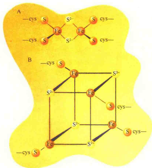
图 7-15 铁硫中心 (引自 Karp, 2010)。A. [2\text{Fe}-2\text{S}] -铁硫中心结构; B. [4\text{Fe}-4\text{S}] -铁硫中心结构。
