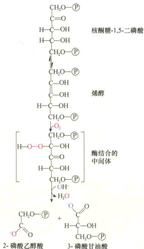
图 8-23 Rubisco 的氧化酶活性 (引自 Nelson and Cox, 2013)。Rubisco 将 \text{O}_2 而不是 \text{CO}_2 添加到核酮糖-1,5 二磷酸上, 形成的中间体极不稳定, 裂解成 3-磷酸甘油酸 (3-phosphoglycerate) 和 2-磷酸乙醇酸 (2-phosphoglycolate)。
