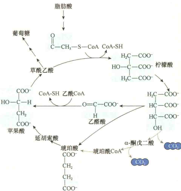
图 8-25 乙醛酸循环 (引自 Cooper and Hausman, 2016)。植物可将脂肪酸经由乙醛酸循环合成糖，是一种改良的三羧酸循环。在乙醛酸循环中，由脂肪酸产生的乙酰 CoA 与草酰乙酸 (oxaloacetic acid) 结合，形成柠檬酸 (citric acid)，柠檬酸进一步转变成异柠檬酸 (isocitrate)，此时的异柠檬酸不需像三羧酸循环那样经过两次脱羧形成琥珀酸 (succinate)，而是直接转变成琥珀酸与乙醛酸。乙醛酸与另 1 分子乙酰 CoA 形成苹果酸，再经草酰乙酸合成糖。
