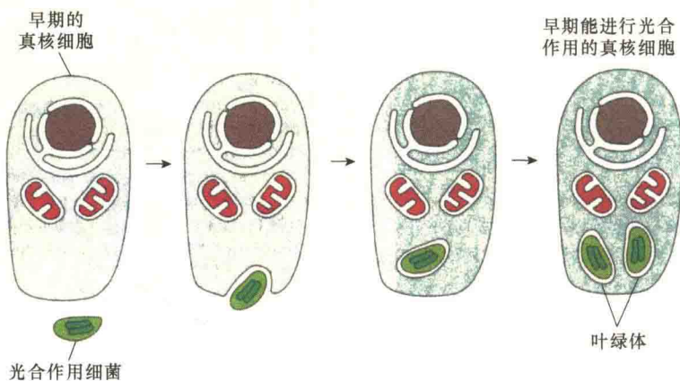
图8-27 叶绿体的起源(引自Alberts et al., 2015)。叶绿体的起源被认为是光合作用细菌与已经含有线粒体的早期真核生物共生而来。
