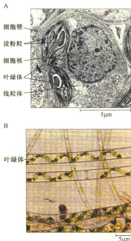
图 8-2 植物细胞中叶绿体的电子显微照片 (引自 Jeff et al., 2012)。A. 植物叶细胞中的叶绿体；B. 海藻细胞中的叶绿体。
