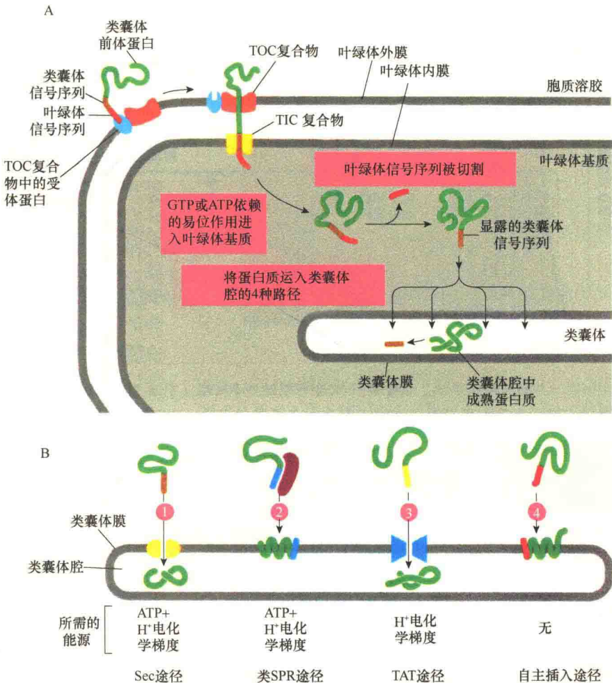
图 8-6 叶绿体前体蛋白转运进入类囊体示意图（引自 Alberts et al., 2015）。A. N 端含有叶绿体信号序列及类囊体信号序列的前体蛋白。首先由叶绿体信号序列引导前体蛋白穿过外膜的 TOC 与内膜的 TIC 进入叶绿体基质，过程与穿过线粒体相似，只不过叶绿体的 TOC、TIC 的组成与线粒体不同。B. 进入叶绿体基质的蛋白质可以通过以下 4 种方式中的一种定位到类囊体的膜或是类囊体腔中：① Sec 途径，即使用的类囊体膜的通道成分是细菌膜通道 Sec 蛋白的同系物；②类 SRP 途径，该途径要借助于 SRP 的同系物；③ TAT（twin arginine translocation）途径，该途径中，信号序列里有两个精氨酸特别关键；④自主插入途径（spontaneous insertion pathway），这一途径可能不需要任何蛋白质的帮助。
