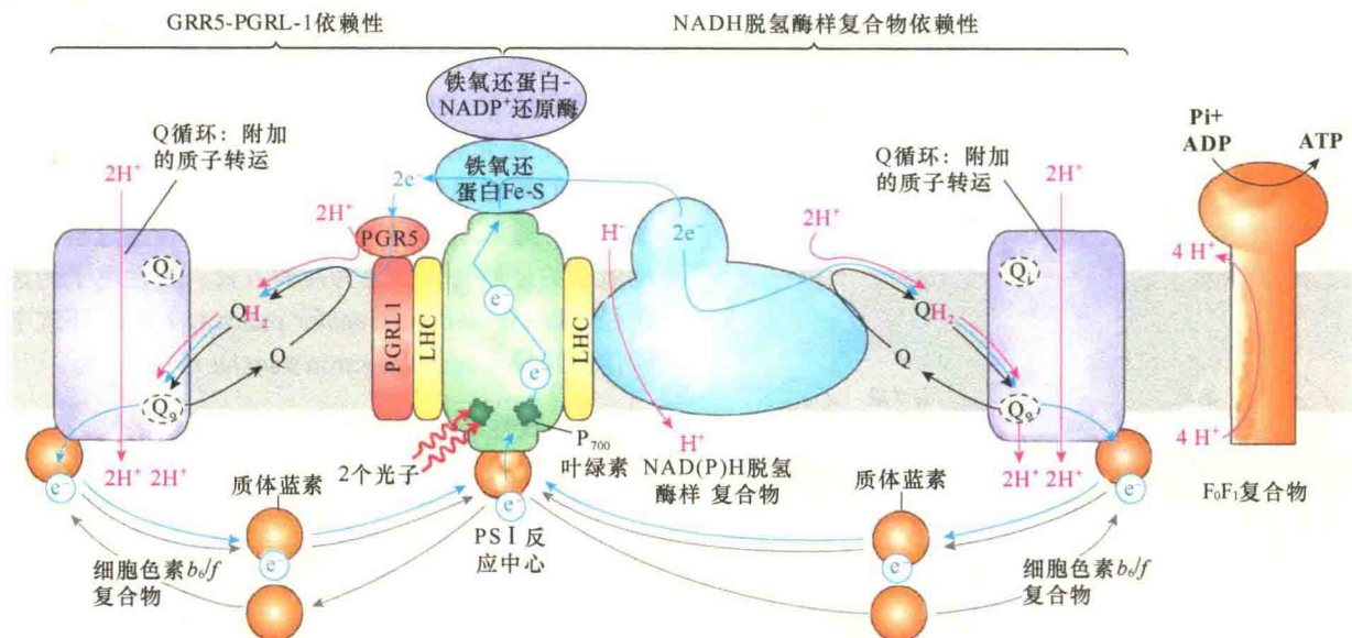
图 8-19 光合作用中循环式电子传递途径 (引自 Lodish et al., 2016)。在循环式电子传递中, 光能被 PS I 用于循环式转运电子从而产生质子动力与 ATP, 而不是用于氧化水及产生 NADPH。高能电子经由 PS I 的铁氧还蛋白或是传递给 PGR5-PGRL1 异源二聚体, 或是传递给 NADH-脱氢酶样复合物, 这两种方式最终都是将质体 Q 还原成 \text{QH}_2 。 \text{QH}_2 又将电子传递给细胞色素 b_6/f , 再传递给质体蓝素, 最后又回到 PS I。
