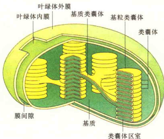
图 8-3 叶绿体的膜与区室 (引自 Wolfe, 1993)。
