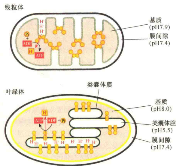
图 8-29 线粒体和叶绿体中 ATP 合酶的定向及 H^+ 的流向 (引自 Alberts et al., 2015)。
