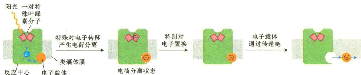
图 8-12 光合反应中心电荷分离简要过程（引自 Alberts et al., 2015）。在反应中心，被捕获的光能用于产生高能电子，这些电子保持在膜的可移动的电子载体中，然后将光能逐渐转变成化学能。当一个光子被反应中心的一对特别的叶绿素分子吸收并将一个电子敲出叶绿素时，即开始了将光能转变成化学能的过程。电子被结合在另一侧膜表面的移动电子载体（橙色）吸收。反应中心内嵌入了一组中间载体，为来自特殊叶绿素对的电子提供传递路径（未显示）。带正电的叶绿素离子与带负电的电子载体之间的物理距离可维持电荷分离状态的短暂稳定，在此期间，叶绿素离子作为强氧化剂，从合适的化合物（如水）中摄取一个电子，然后电子载体扩散离开反应中心，成为一个强大的电子供体，将其电子转移到电子传递链上。
