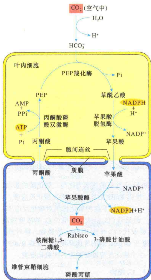
图 8-24 \text{C}_4 植物碳的固定 (引自 Nelson and Cox, 2013)。在 \text{C}_4 植物中, 卡尔文循环发生在维管束鞘细胞, 位于组织的内层。 \text{C}_4 植物利用叶肉细胞固定 \text{CO}_2 , 然后在维管束鞘细胞中释放, 保证了 \text{CO}_2 高浓度进入卡尔文循环。
