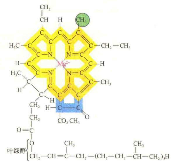
图 8-9 叶绿素 a 的结构（引自 Lodish et al., 2016）。
