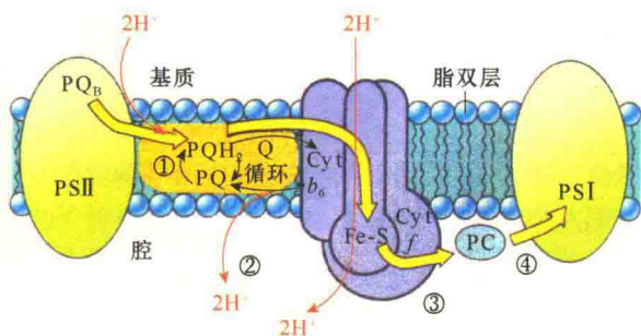
图 8-17 电子在 PS II 与 PS I 之间的传递（引自 Karp, 2010）。
