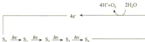
图 8-16 Mn 的电子传递与水的光解 (引自 Karp, 2010)。S 表示 Mn 基团的正电荷数。
