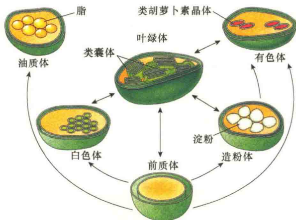
图 8-1 前质体的分化途径 (引自 Cooper and Hausman, 2016)。
