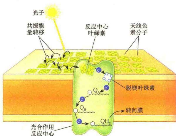
图 8-11 光合中心的组织结构及激发能转移（引自 Cooper and Hausman, 2013）。光合中心（photocenter）由几百个天线色素分子构成，它们吸收光子并将光能转移给中心叶绿素。反应中心叶绿素将激发的电子传递给电子传递链中的受体——脱镁叶绿素（pheophytin），从而将高能电子转运进入电子传递链。
