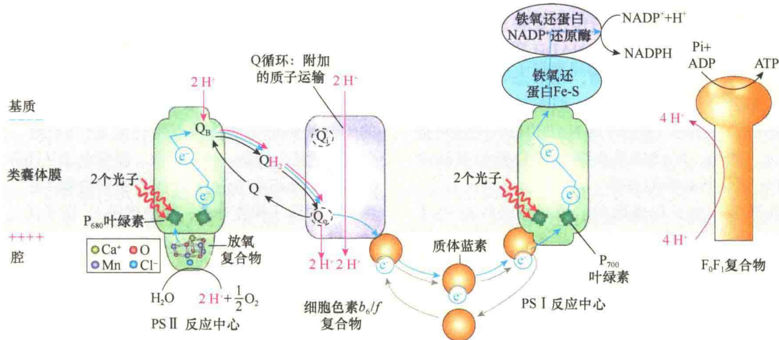
图 8-18 光合作用中线性电子传递途径（引自 Lodish et al., 2013）。在非循环式电子传递途径中，电子的最终受体是 \text{NADP}^+ ，电子供体来自光解的水。
