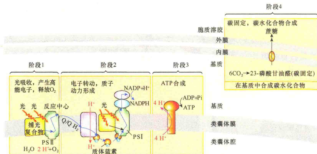
图 8-7 光合作用的四个阶段 (引自 Lodish et al., 2016)。
