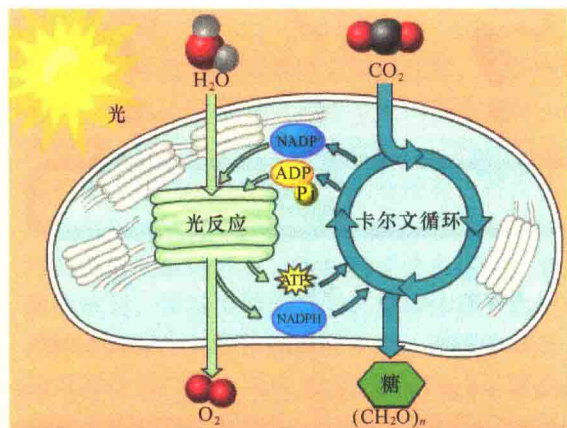
图 8-8 光合作用的两个阶段：光反应与暗反应。
