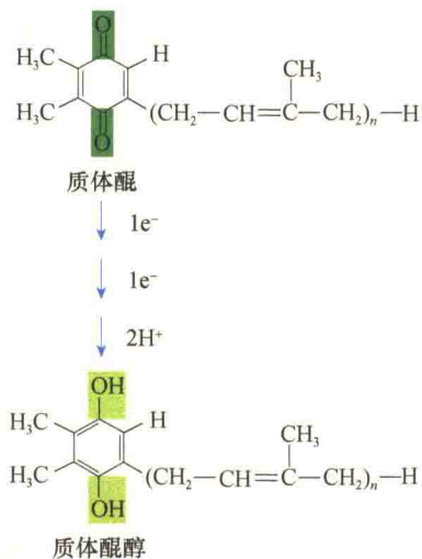
图 8-14 质体醌的氧化和还原状态 (引自 Karp, 2010)。
