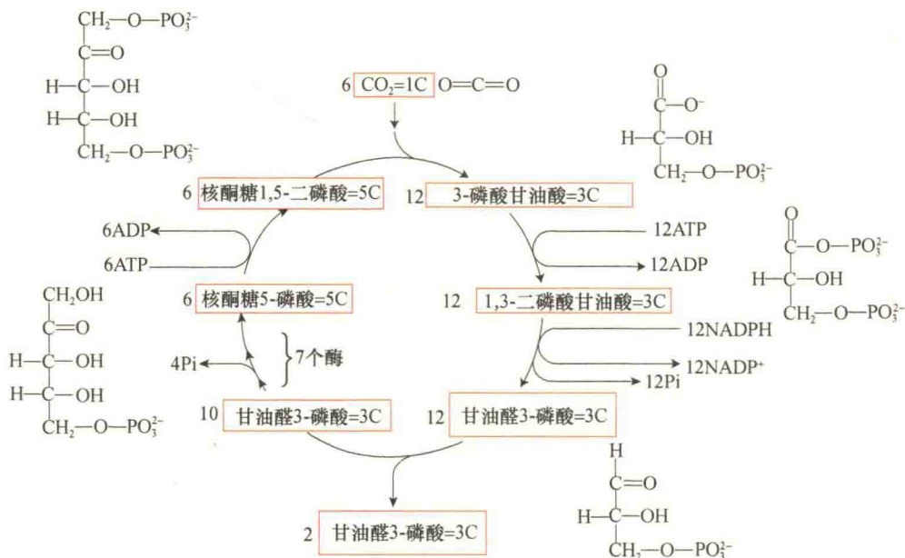
图 8-22 卡尔文循环 (改自 Lodish et al., 2013)。
