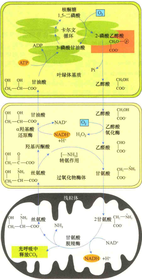
图 8-26 过氧化物酶体在光呼吸中的作用 (引自 Nelson and Cox, 2013)。在光合作用期间，CO 2 经卡尔文循环被转变成糖，反应的第一步是将 CO 2 添加到五碳糖——核酮糖 1,5-二磷酸上。但是，起催化反应的酶有时会错误地将 O 2 分子而不是 CO 2 添加到核酮糖 1,5-二磷酸上，这样产生的产物是二碳的磷酸乙醇酸 (phosphoglycolate)，磷酸乙醇酸可转变成乙醇酸 (glycolate)，并被转移到过氧化物酶体，在过氧化物酶体中被氧化转变成甘氨酸。随后，甘氨酸被转移到线粒体，并在线粒体中转变成丝氨酸。丝氨酸又重新回到过氧化物酶体，并转变成甘油酸 (glycerate)。
