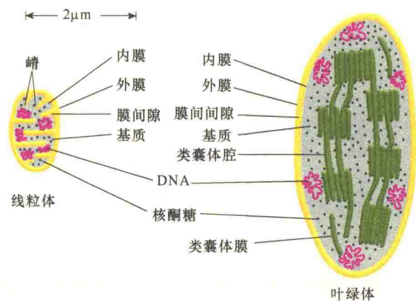
图 8-28 叶绿体与线粒体的比较 (Alberts et al., 2015)。线粒体和叶绿体的膜及区室在结构组成和功能上都有所不同, 如线粒体内膜除了作为线粒体界膜之外, 主要功能是电子传递和合成 ATP。从结构上看, 线粒体内膜向内折叠成嵴, ATP 合酶位于嵴上。而叶绿体的内膜只是稍向内折形成小管或小泡结构, 且表面光滑。叶绿体内膜是脂合成的场所, 是叶绿体的界膜。
