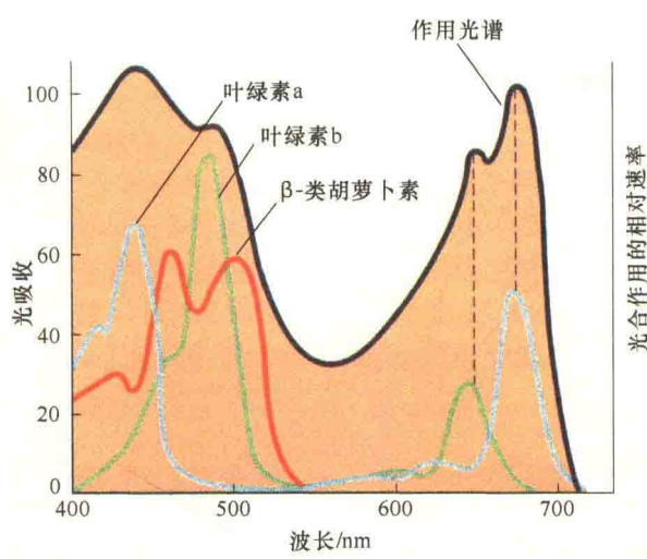
图 8-10 光合作用的作用光谱（引自 Lodish et al., 2016）。图中的作用光谱是指不同波长光对植物叶光合作用的影响；吸收光谱是三种色素联合起来的吸收光谱，三种不同色素的吸收光谱用不同颜色的线表示。
