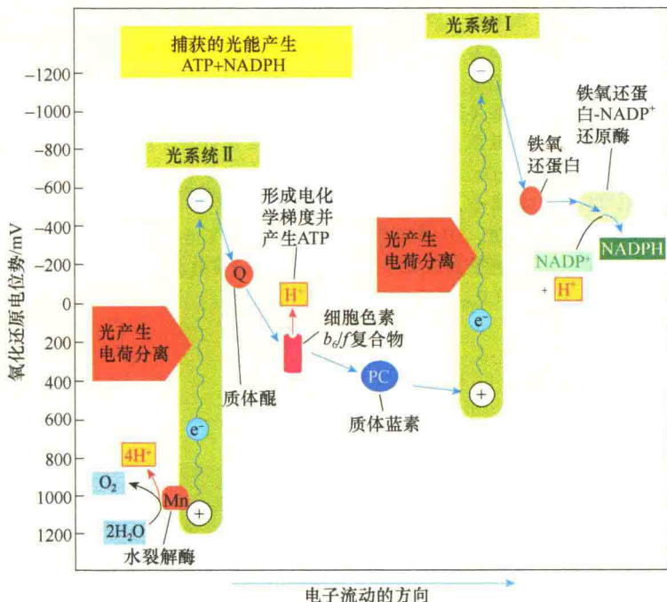
图8-13 光合作用中的Z形电子传递链及氧化电势的变化(引自 Alberts et al., 2015)。该传递链中除了水、PS II、PS I外,还有质体醌、质体蓝素、细胞色素 b_6/f 、Fd等。由于各电子载体在电子传递链中的氧化电势的不同,呈现Z字形。PS II将来自水的电子传递给PS I,而PS I则通过铁氧还蛋白-NADP + 还原酶(ferredoxin-NADP + reductase)传递给NADP + 。净电子流是两个光系统协同将来自水的电子流向NADP + ,同时产生了NADPH及电化学质子梯度。形成的质子梯度可用于ATP的合成。
