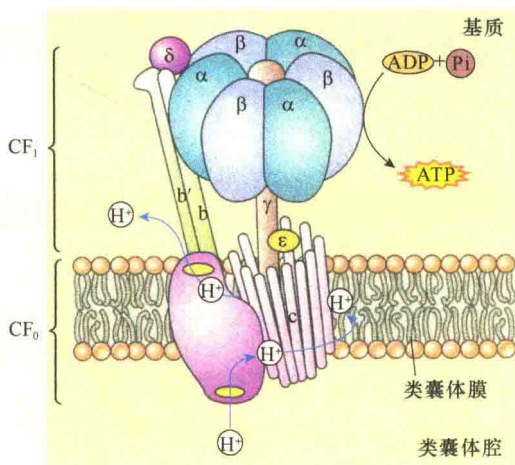
图 8-20 叶绿体 CF_0 - CF_1 ATP 合酶结构示意图 (引自 Taiz and Zeiger, 2015)。
