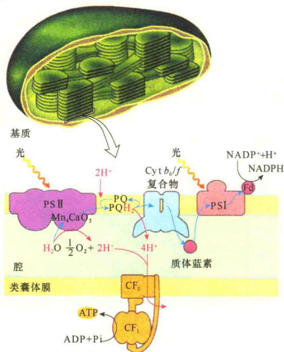
图 8-21 光合磷酸化与质子、电子回路 (引自 Nelson and Junge, 2015)。
