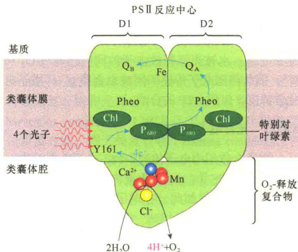
图 8-15 PS II 中的电子流与氧的产生 (引自 Lodish et al., 2013)。PS II 反应中心含有两个整合蛋白质, 分别称为 D1 和 D2, 以及一对特别的叶绿素 ( \text{P}_{680} )。在该反应中心的类囊体腔面膜上结合着一些电子载体, 形成放氧复合物。在放氧复合物中另有 3 个外在蛋白质 (相对分子质量为 33kDa、23kDa 和 17kDa)、4 个锰离子、1 个钙离子、1 个氯离子, 这些离子参与 \text{H}_2\text{O} 的裂解、维持环境中 \text{O}_2 的高比值。D1 多肽中的酪氨酸 161 (Y161) 可促进 Mn 产生的电子去氧化反应中心的叶绿素 ( \text{P}_{680}^+ ), 使之还原到基态 ( \text{P}_{680} )。
