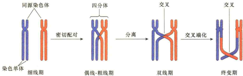
图 13-57 同源染色体联会时的交换和交叉（引自 Kleinsmith and Kish, 1995）
