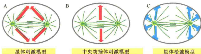
图 13-50 胞质分裂收缩位点确定的三种可能机制 (引自 Alberts et al., 2015)。图中显示的是后期纺锤体微管产生的信号对收缩位置影响的三种现代模型。需要说明是, 任何单一的模型都不能解释所有观察到的现象, 或许卵裂沟的确定需要这三种模型共同作用。
