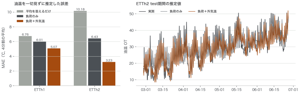
外気温を足すとETTh2の油温推定はMAE 3.2℃、平均予測の3分の1になる
