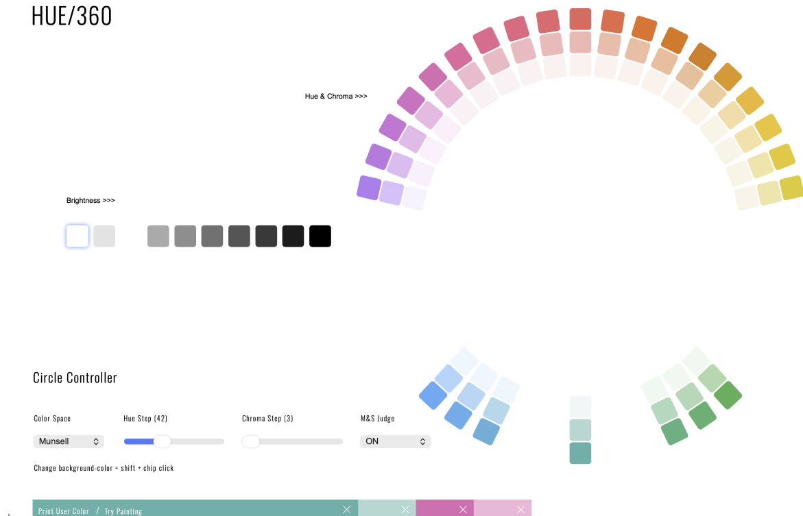
図 D.10: Hue360
