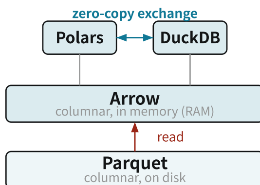
図 5.3: Parquet と Arrow
