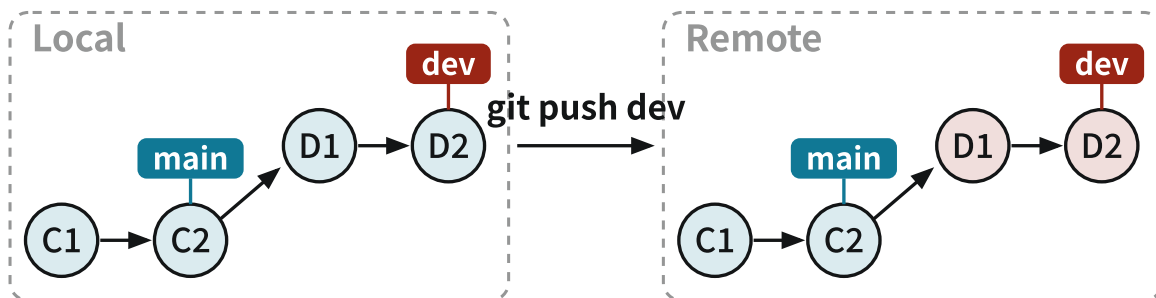
図 3.19: dev を push
