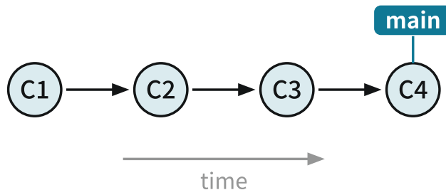
図 3.3: コミット
