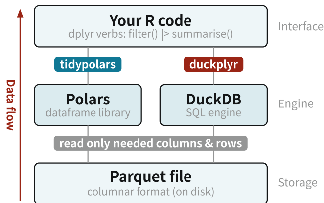
図 5.1: Parquet・Polars・DuckDB の関係
