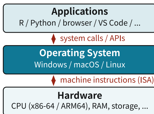
図 1.7: ハードウェア, OS, アプリケーションの階層
