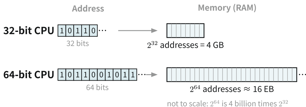
図 1.6: アドレス幅と扱えるメモリの上限
