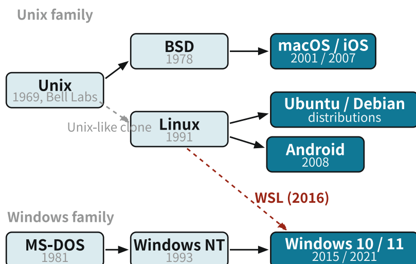
図 1.8: OS の系譜
