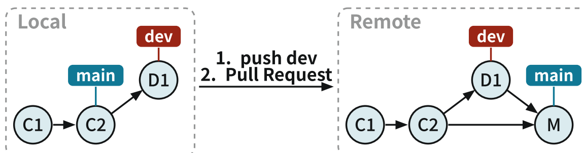
図 3.13: リモートマージ (Pull Request)
