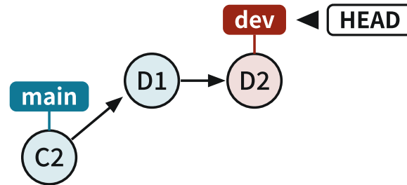
図 3.18: コミットを積む
