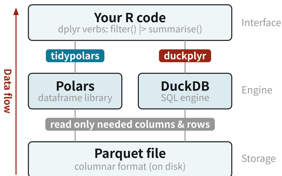
図 5.1: Parquet・Polars・DuckDB の関係
