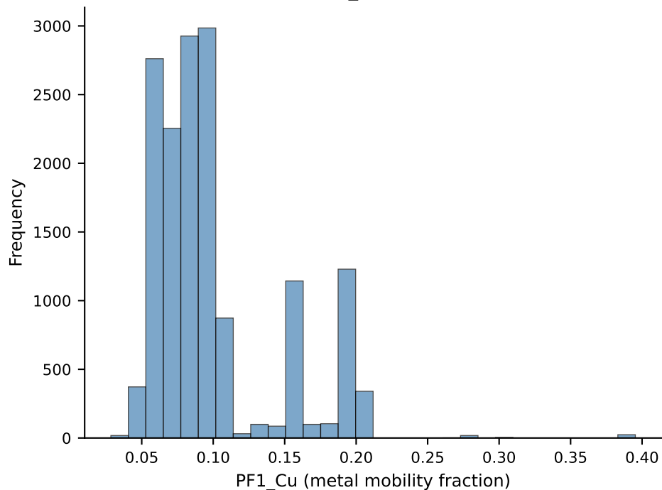
SPIRE PF1_Cu (n=15368)
