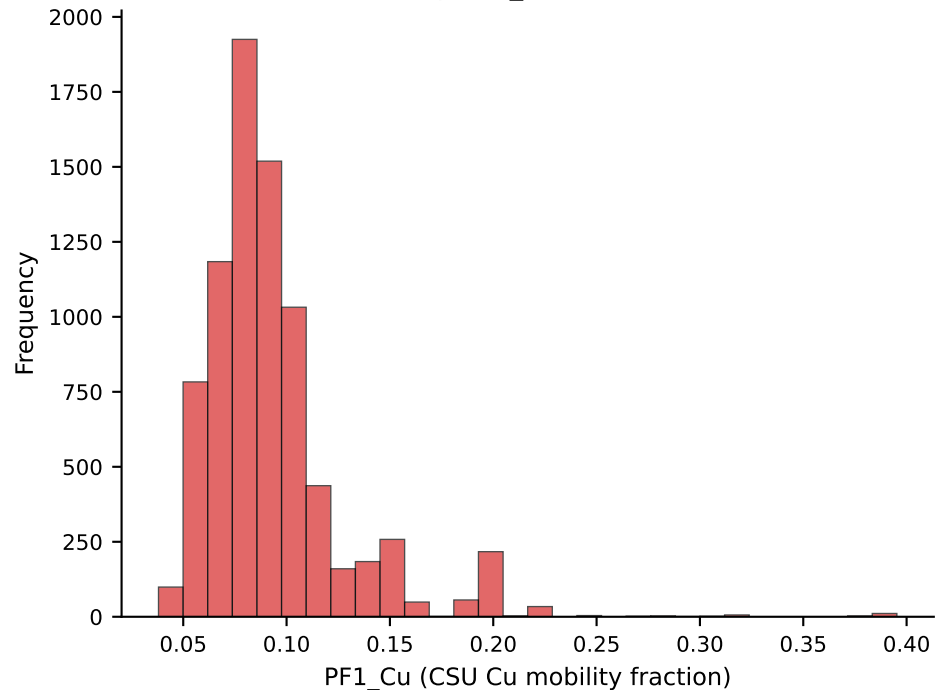
MGnify PF1_Cu (n=7973)
