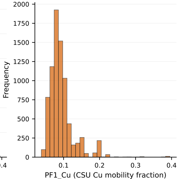
MGnify PF1_Cu (n=7973)
