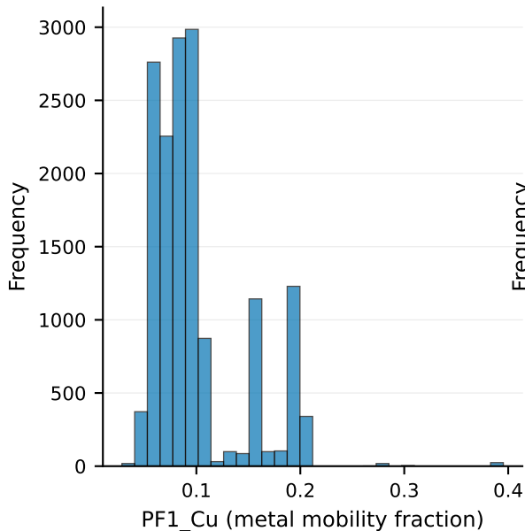
SPIRE PF1_Cu (n=15368)
