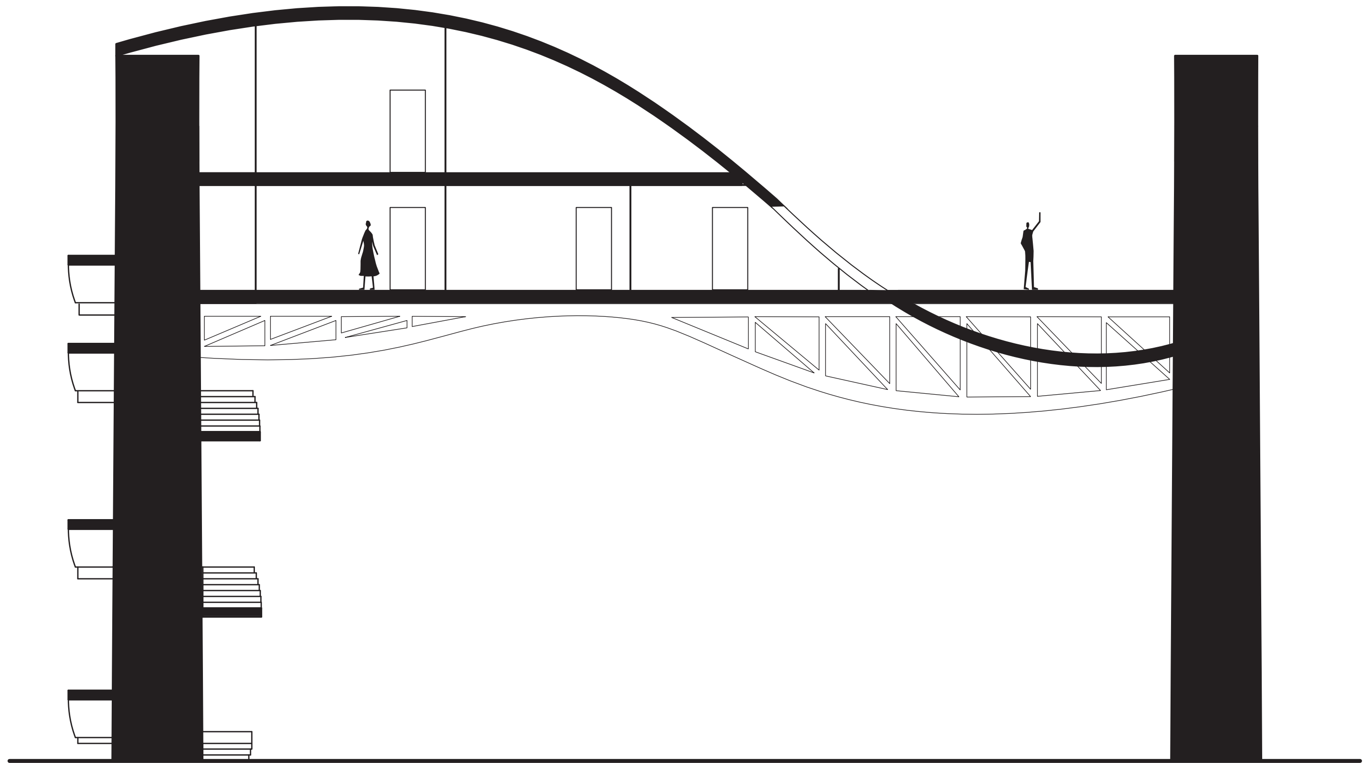
SECTION B SCALE: 1/8"=1'-0"
