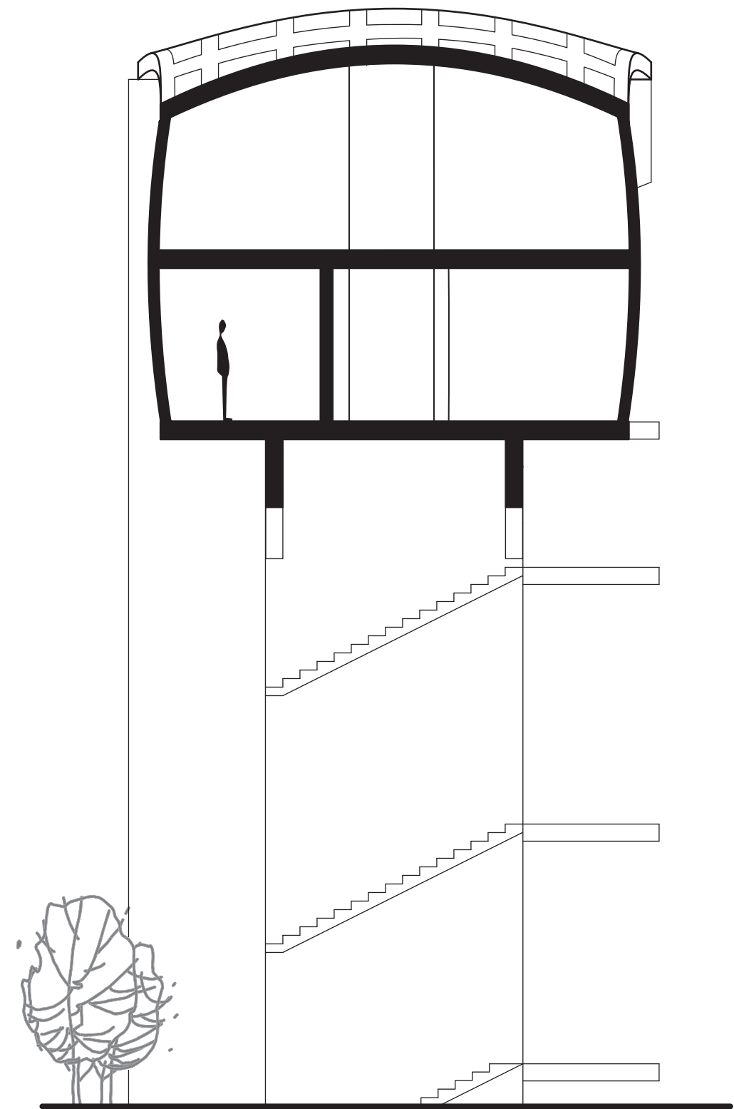
SECTION A SCALE: 1/8"=1'-0"
