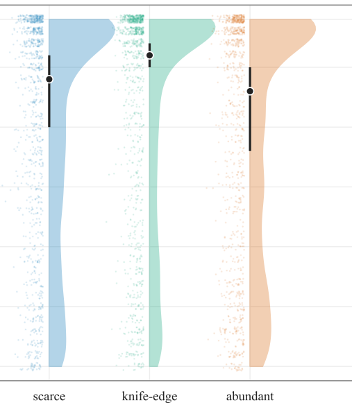
L3 · association
