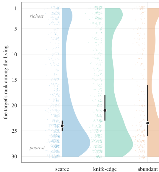
L2 · predation
