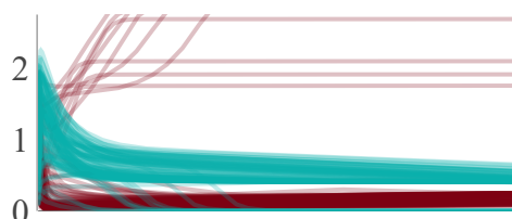
D. Parameter Variation: Healthy
