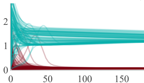
D. Parameter Variation: Healthy
