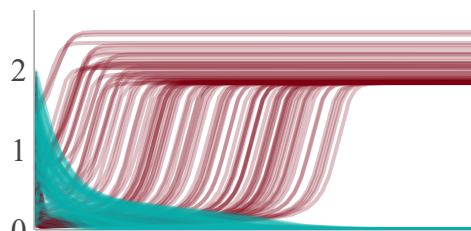
C. Parameter Variation: Bistability
