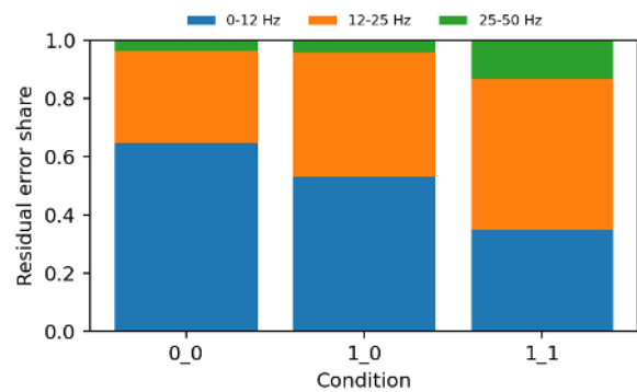
[그림7: 조건별 대역 재구성 오차 기여도]
