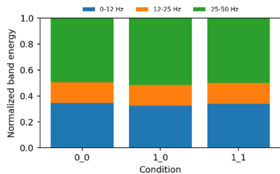
[그림9: 조건별 주파수 대역 에너지 분포]
