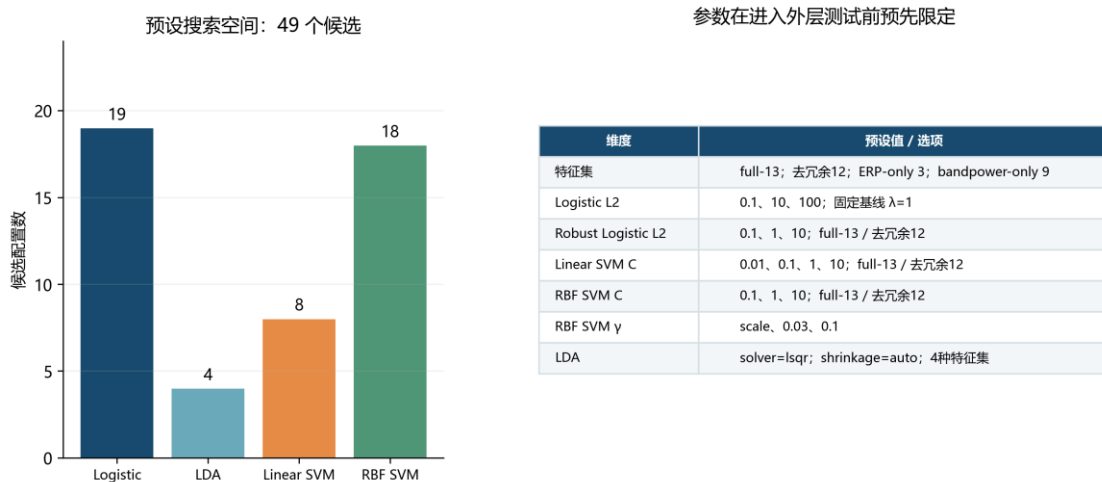
图7 候选分类特征网格
