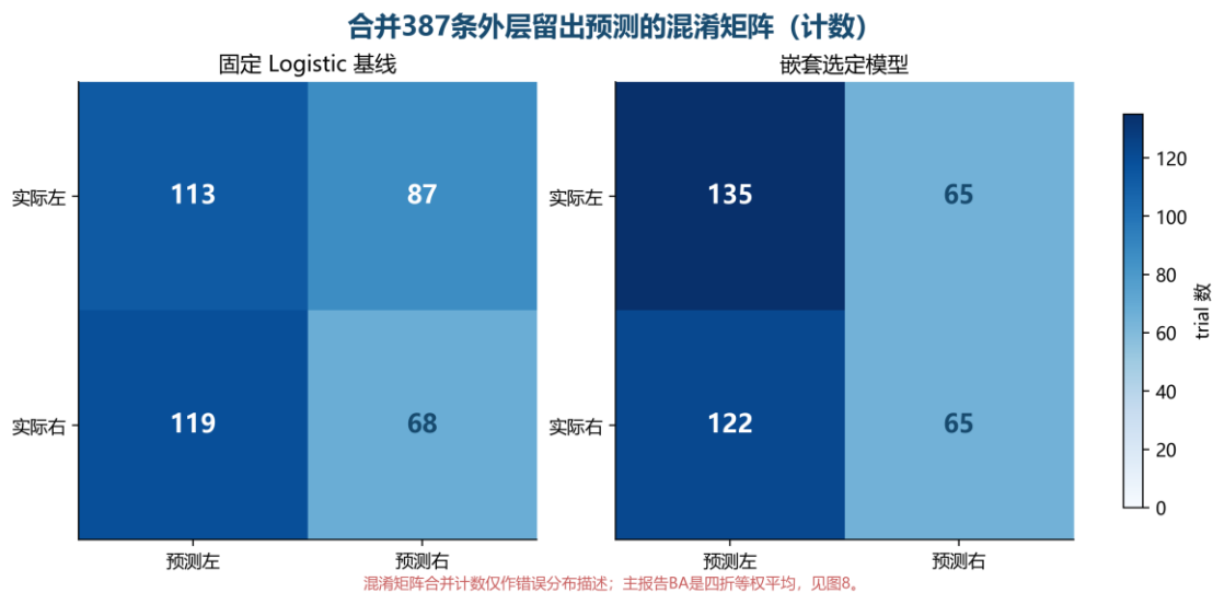
图10 留出记录混淆矩阵
