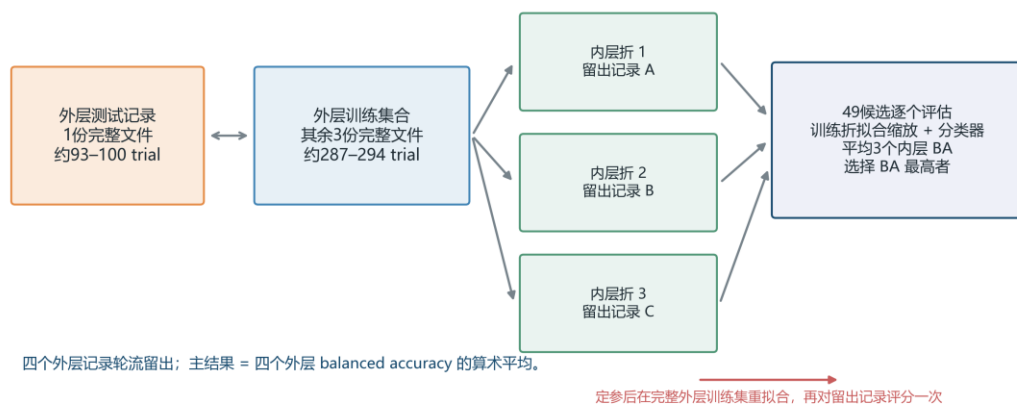
图8 固定主模型的嵌套/分组验证示意
