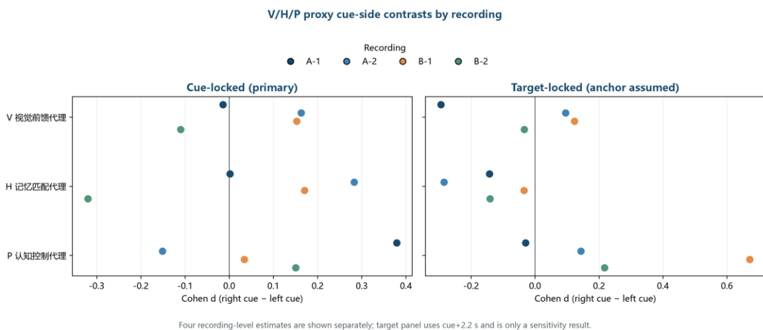
图11 状态代理量的记录间效果
