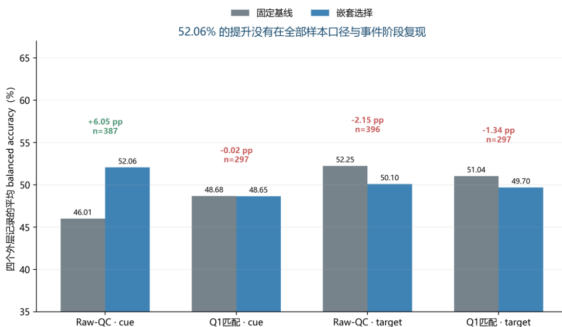
图 12 分析样本和验证范围敏感性
