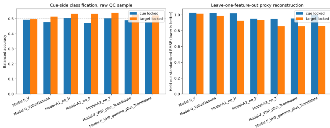
图13 V/H/P 消融效应
