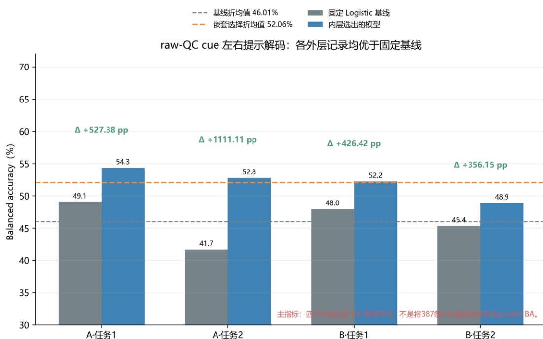
图9 主模型结果汇总
