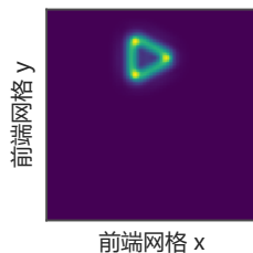
右 cue: Gabor 能量 (100 ms)
