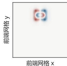
右 - 左 Gabor 能量
