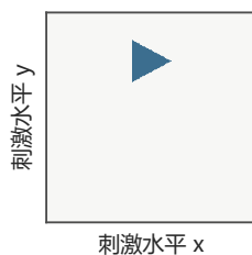
右 cue-圆形基线
