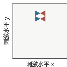
右-左 (基线相减后)
