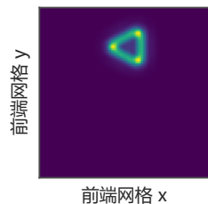
左 cue: Gabor 能量 (100 ms)
