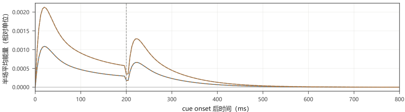
按视觉半场汇总的空间 Gabor 能量
