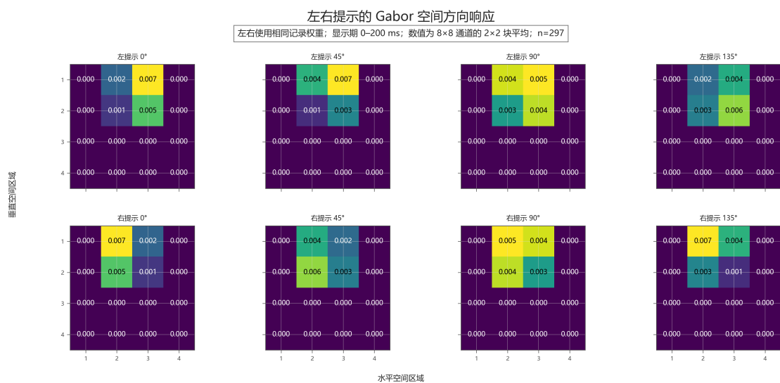
图 6 左右提示的 Gabor 空间方向响应。行表示提示方向，列表示滤波方向；每个数值为原生 8 \times 8 空间通道相邻 2 \times 2 块的均值，四个方向分别展示而未合并；同一方向下左右使用相同色标，不同方向之间不比较颜色幅度。
