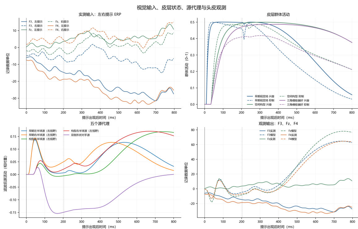
图 7 视觉输入、皮层状态、源代理与头皮观测
