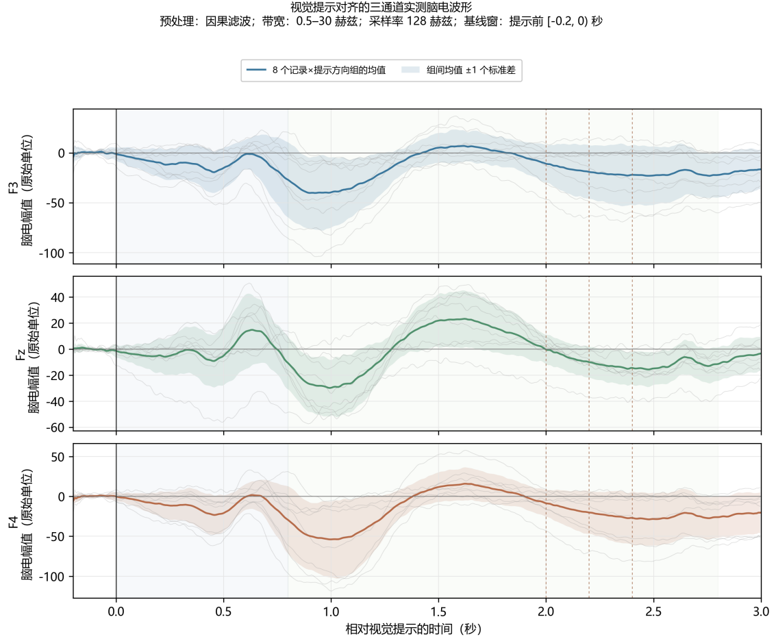
图 2 F3、Fz、F4提示对齐波形
