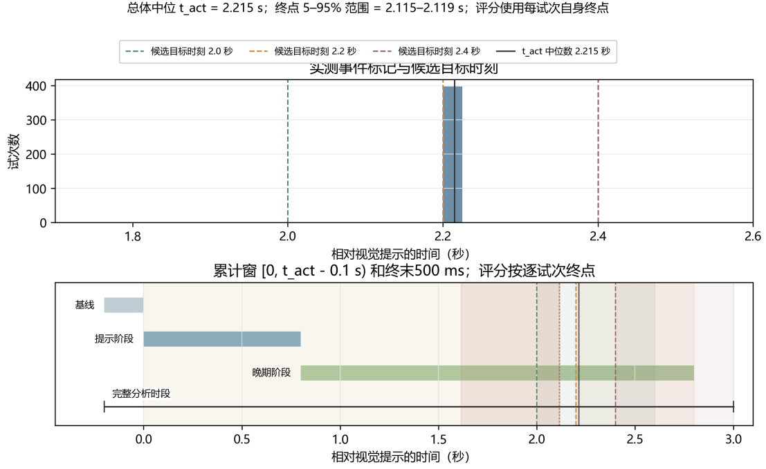
图 1 事件标记与分析窗
