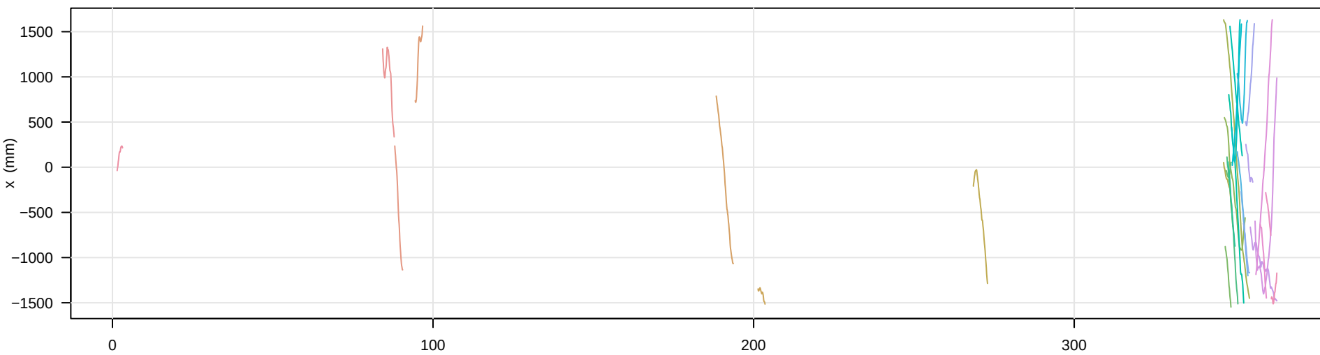
Anopheles coluzzii ... real trajectories (x, y, z vs time)
