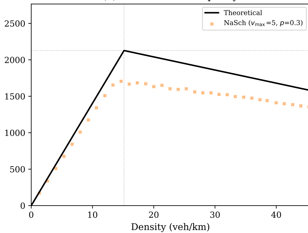
(d) NaSch — near capacity
