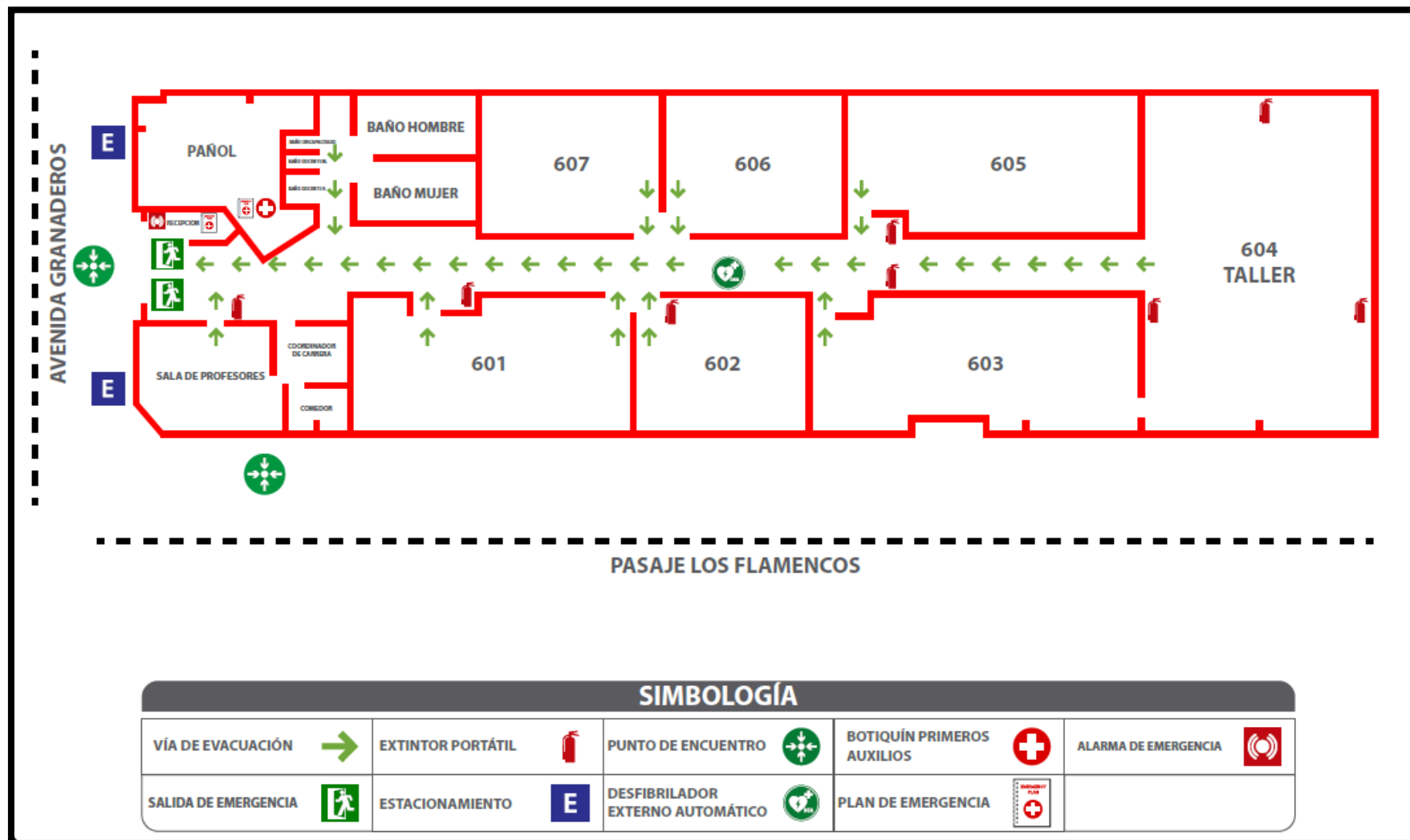
Imagen VII. Plano Evacuación Subsede Maquinaria Pesada.
