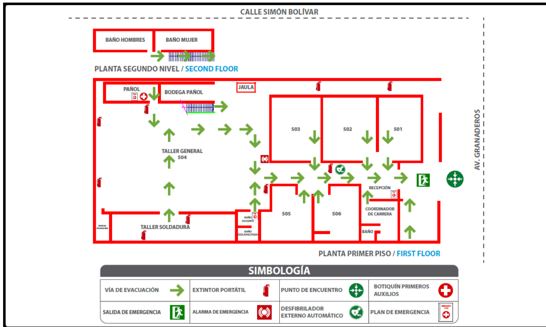
Imagen VI. Plano Evacuación Subselección Mantenimiento Plantas Mineras.
