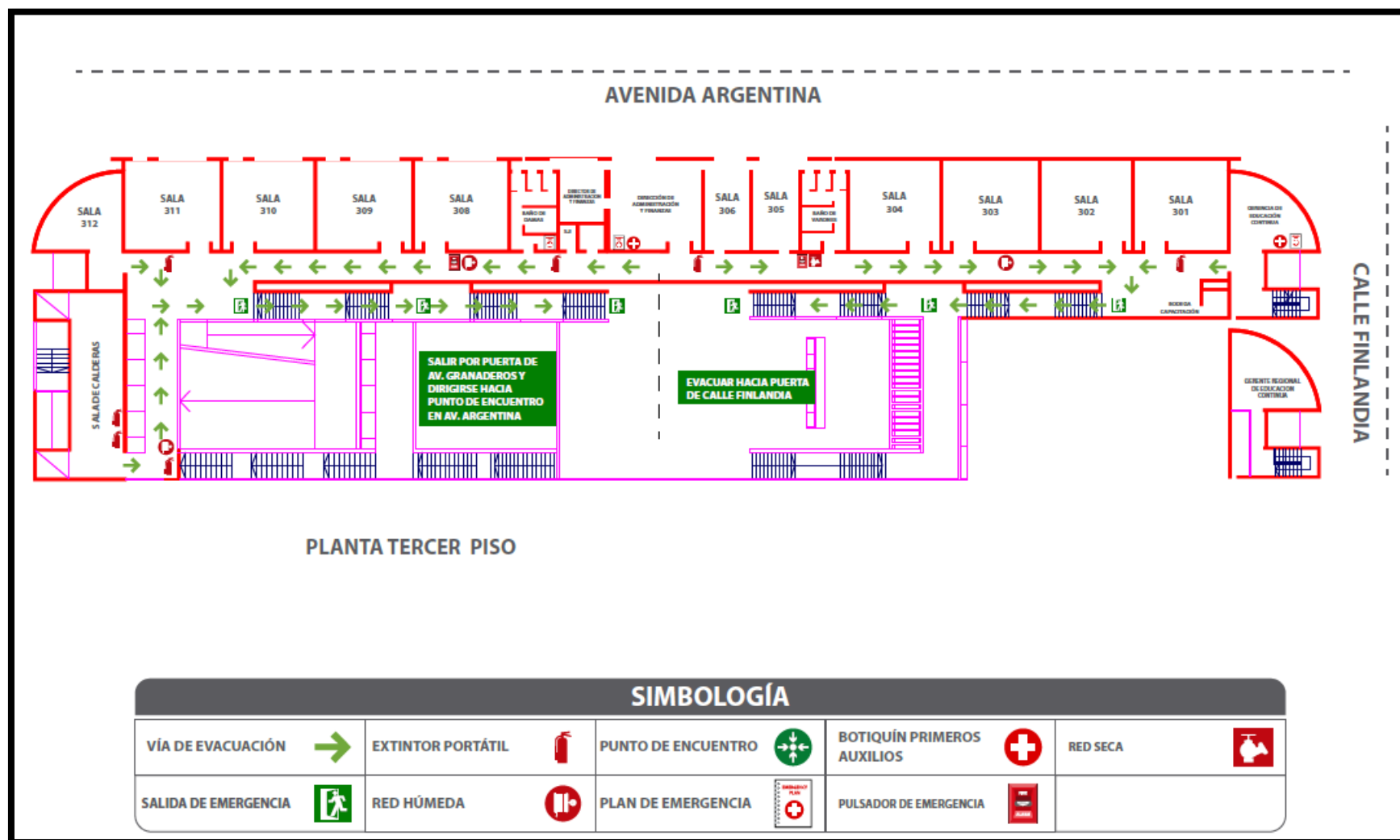
Imagen III. Plano Evacuación Sede Principal – Tercer Piso.
