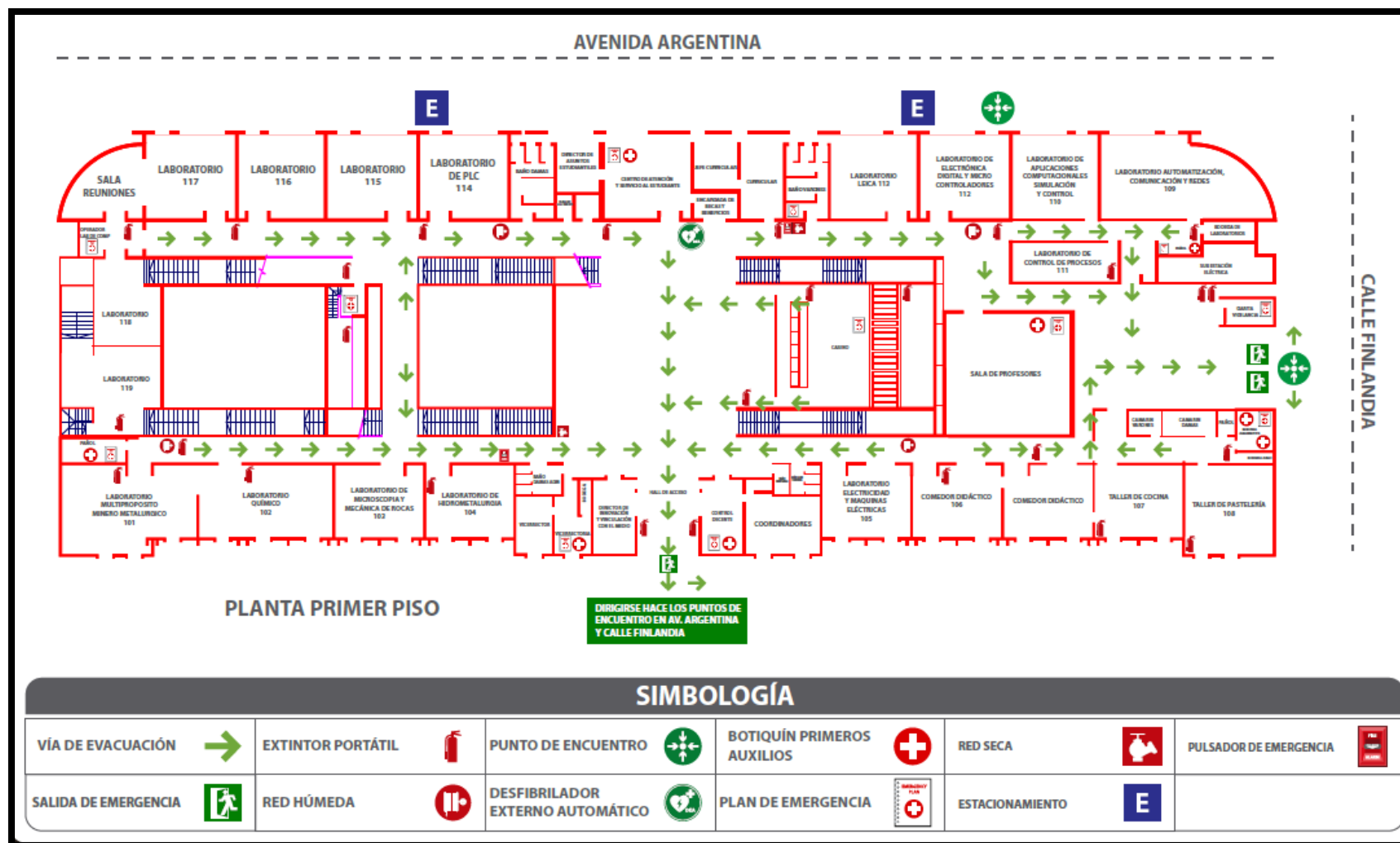
Imagen 1. Plano Evacuación Sede Principal – Primer Piso.
