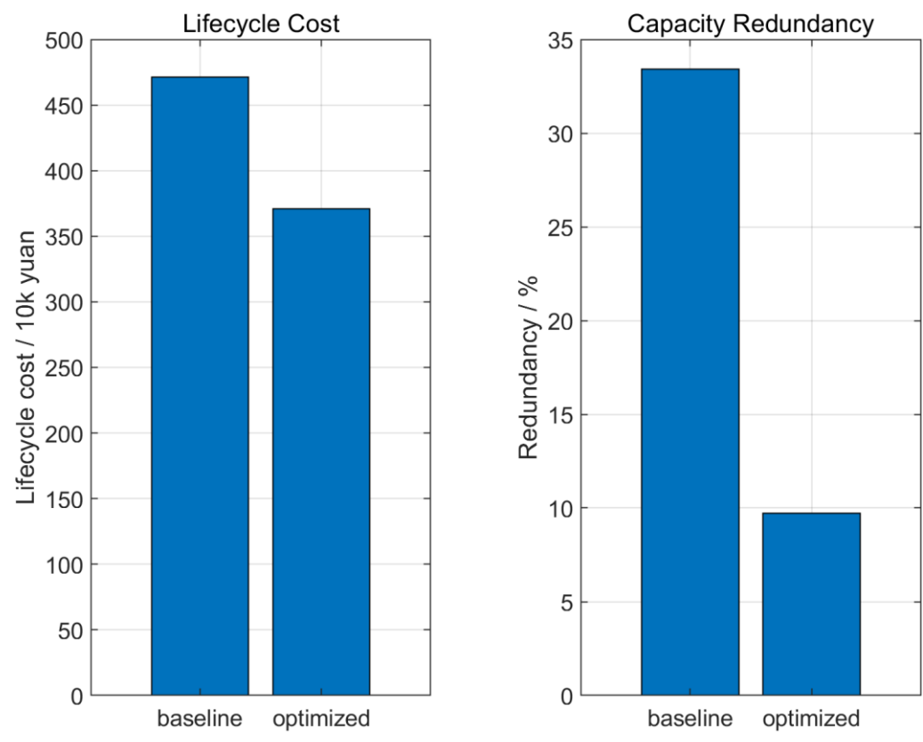
【图 6-1 基准方案与优化方案对比图】
