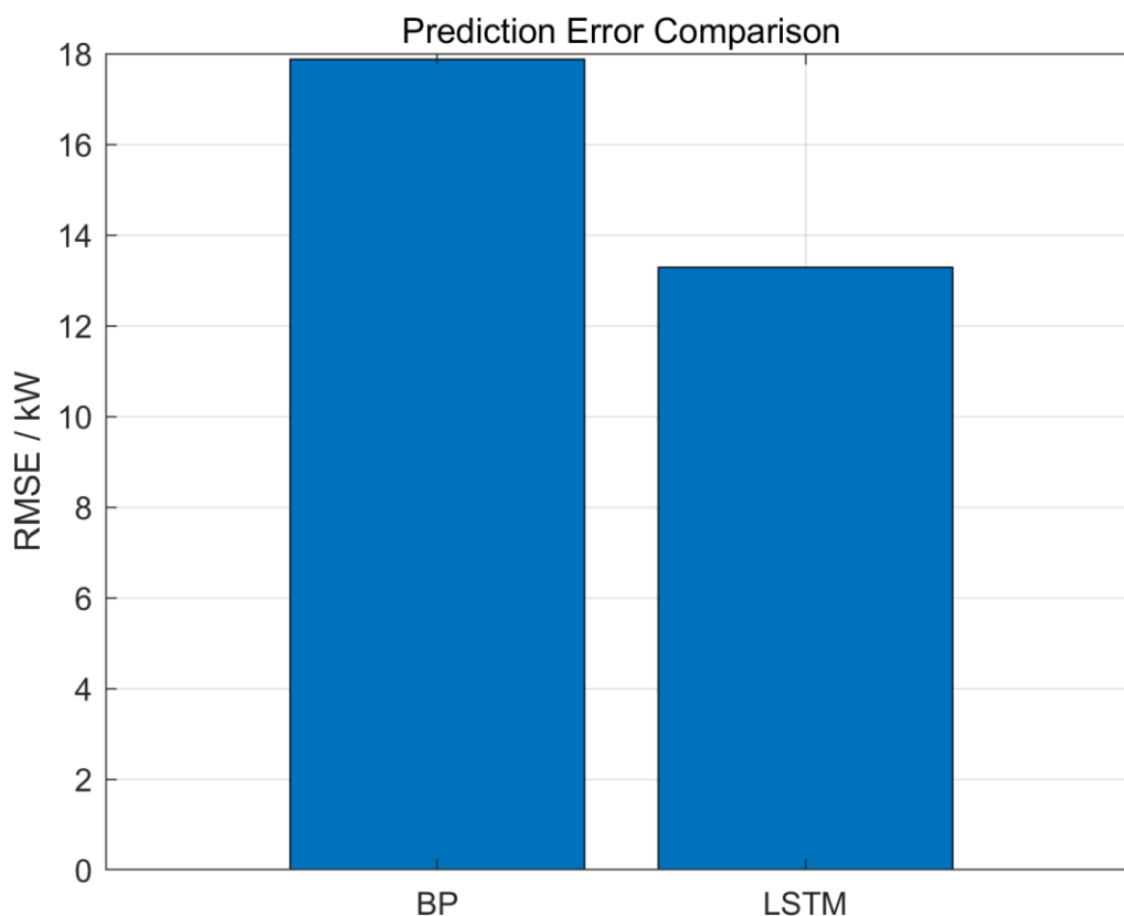
【图 4-5 模型 RMSE 对比图】
