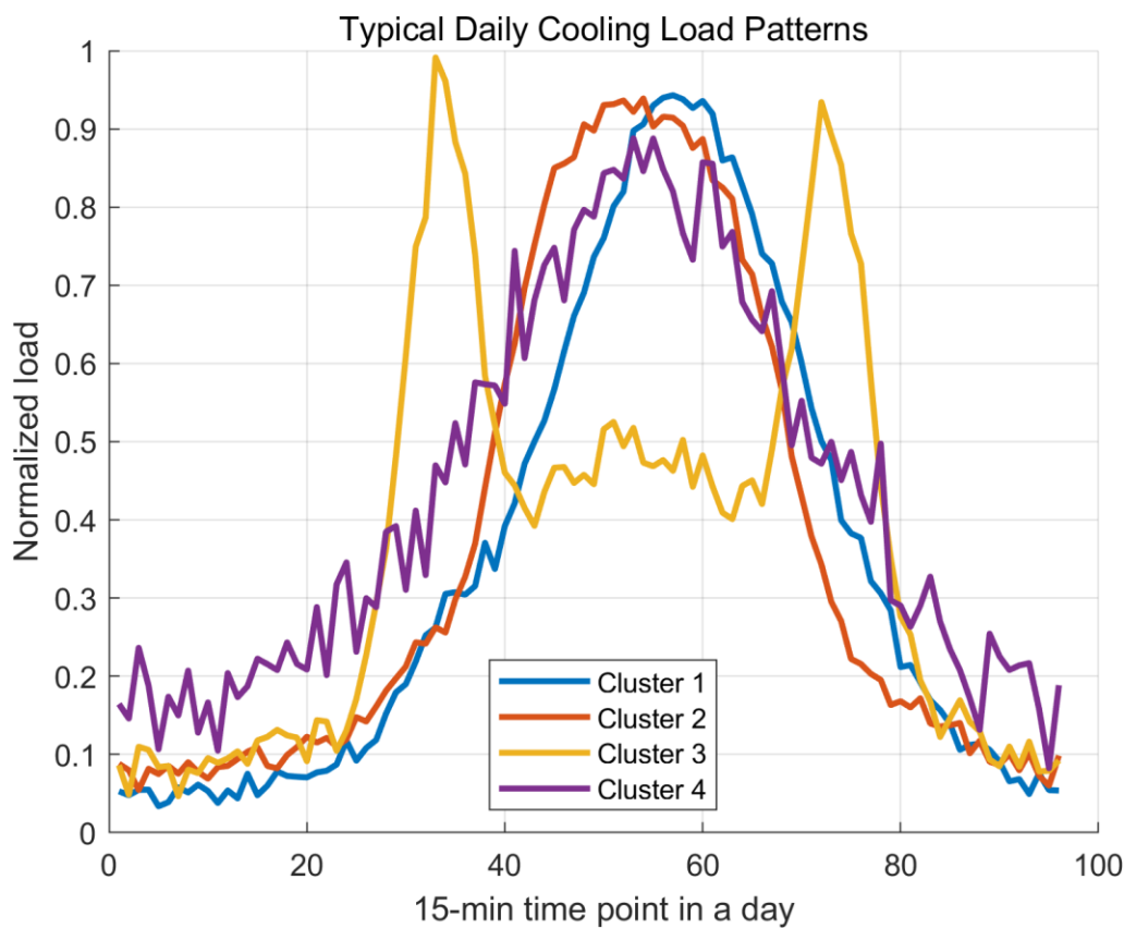
【图 3-6 典型日负荷曲线聚类图】
