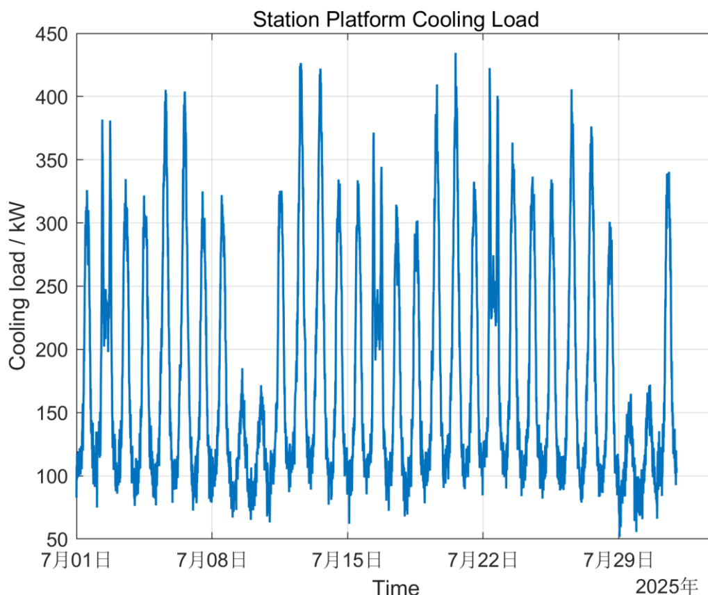
【图 3-3 站台总冷负荷时间序列图】
