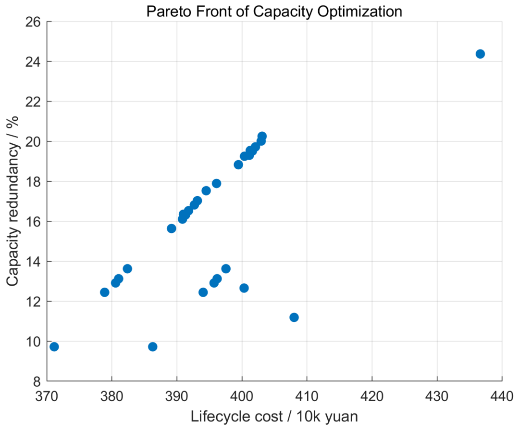
【图 5-2 Pareto 前沿图】
