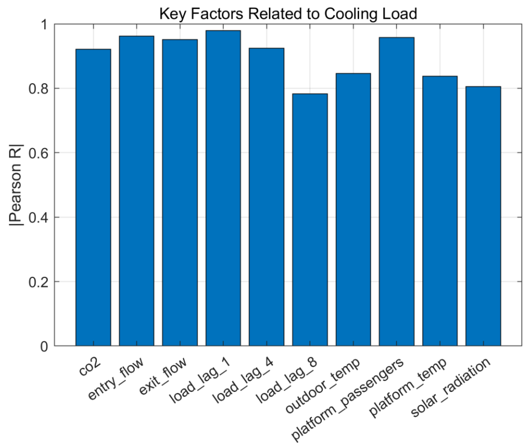
【图 3-4 Pearson 相关性排序图】
