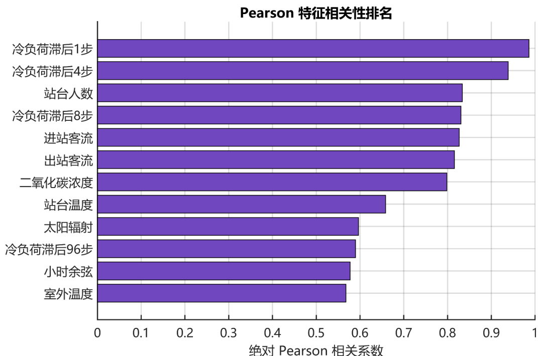
图 3-3 Pearson 相关性排序图
