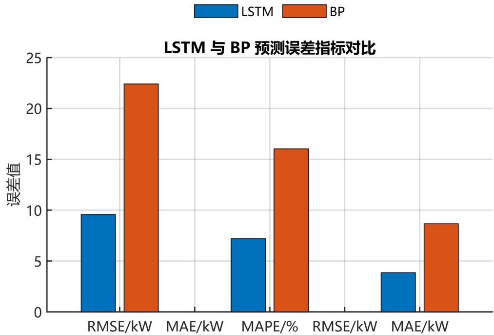
图 4-6 LSTM 与 BP 预测误差指标对比图
