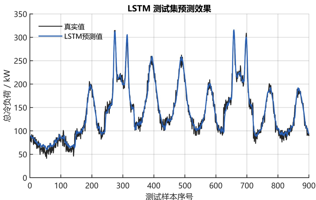
图 4-4 LSTM 测试集预测结果图
