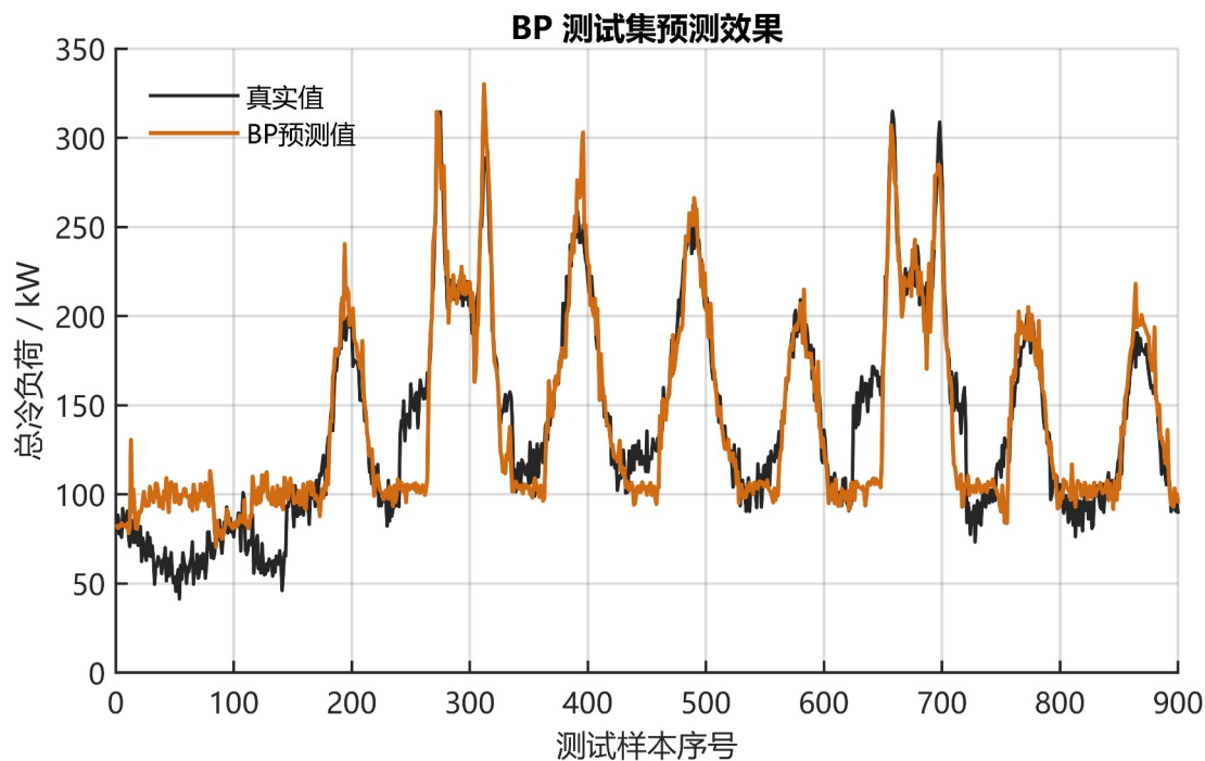
图 4-5 BP 测试集预测结果图
