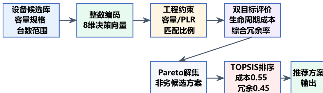
图 5-1 NSGA-II 与 TOPSIS 容量优化流程图
