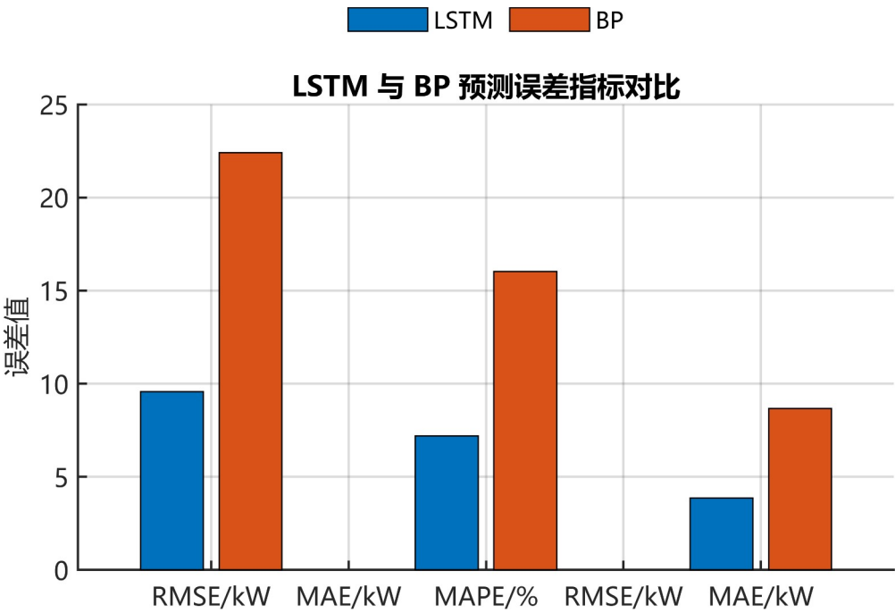
图 4-6 LSTM 与 BP 预测误差指标对比图
