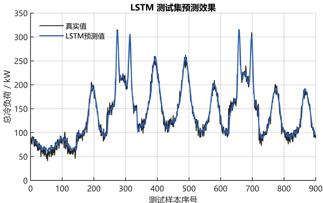
图 4-4 LSTM 测试集预测结果图
