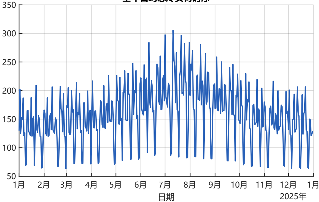
全年日均总冷负荷时序
