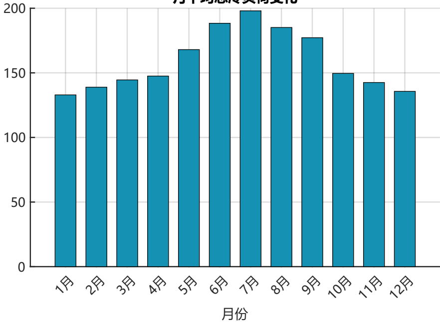
月平均总冷负荷变化
