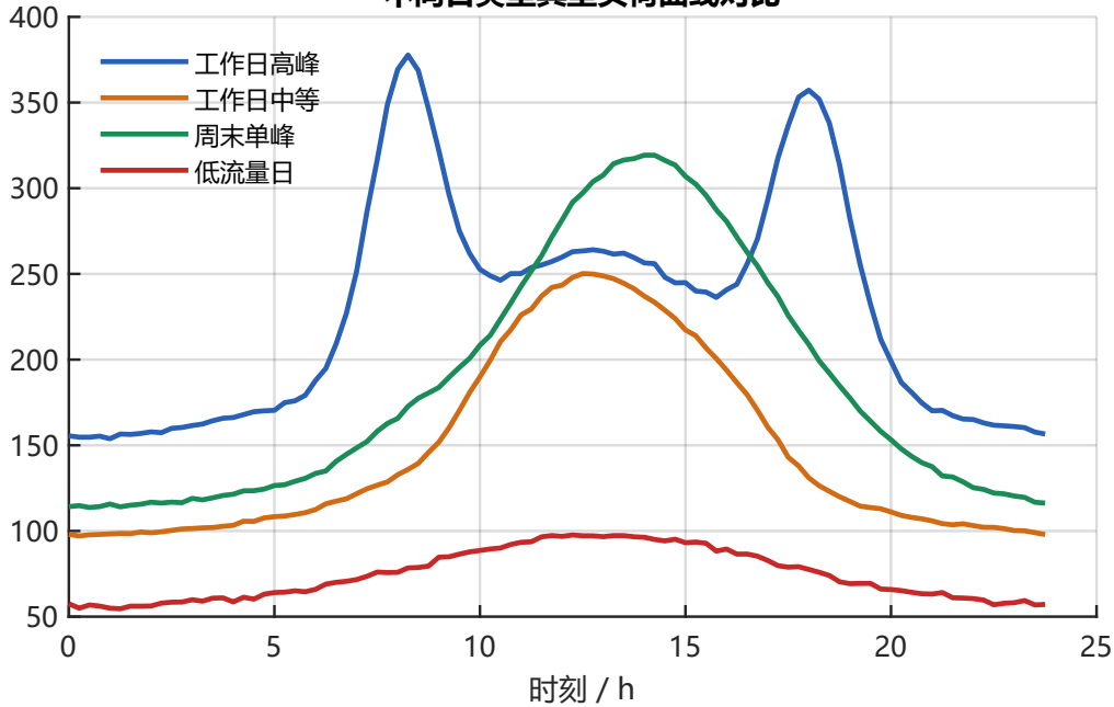
不同日类型典型负荷曲线对比
