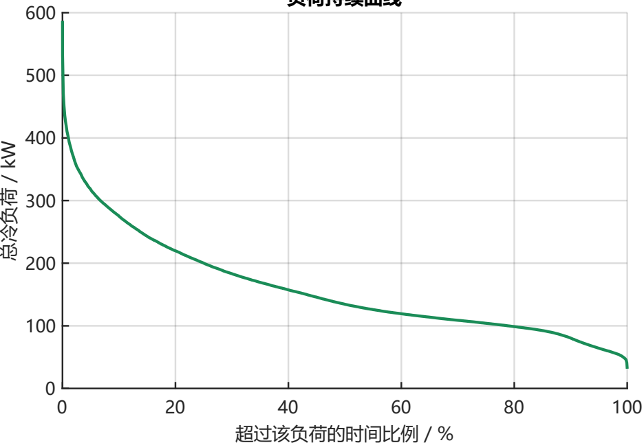
负荷持续曲线
