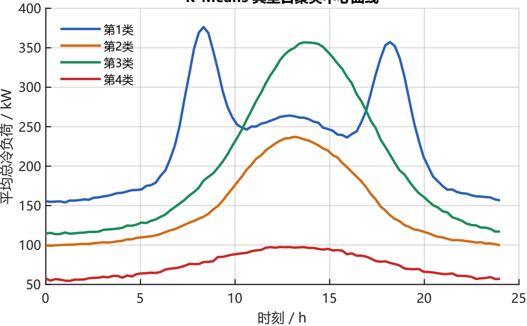
K-Means 典型日聚类中心曲线
