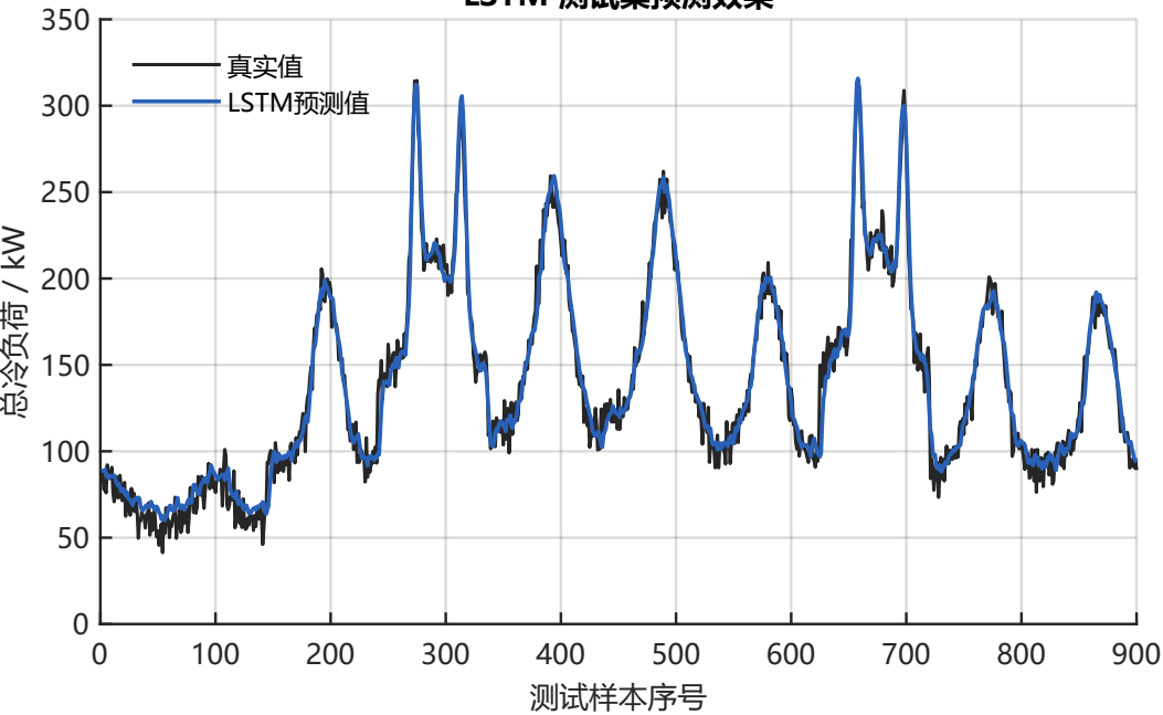
LSTM 测试集预测效果
