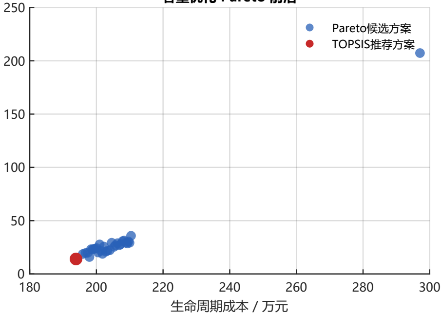
容量优化 Pareto 前沿
