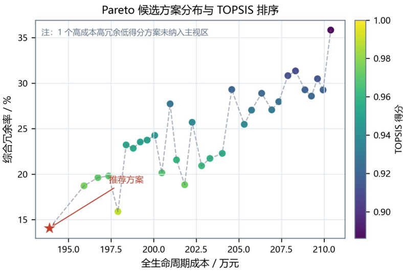
图 5-2 Pareto 前沿图
