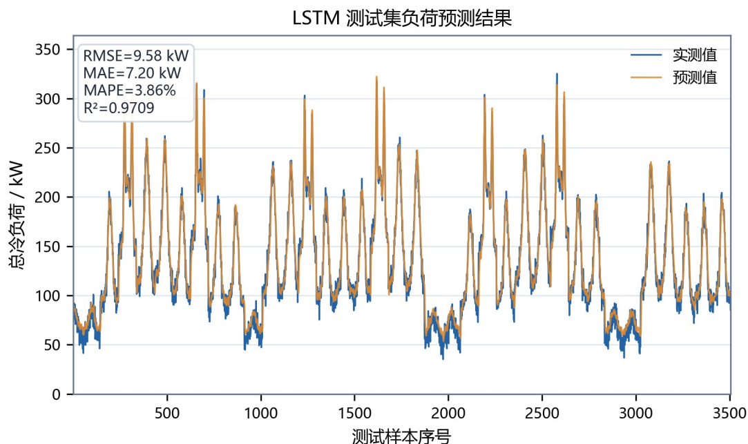
图 4-4 LSTM 测试集预测结果图
