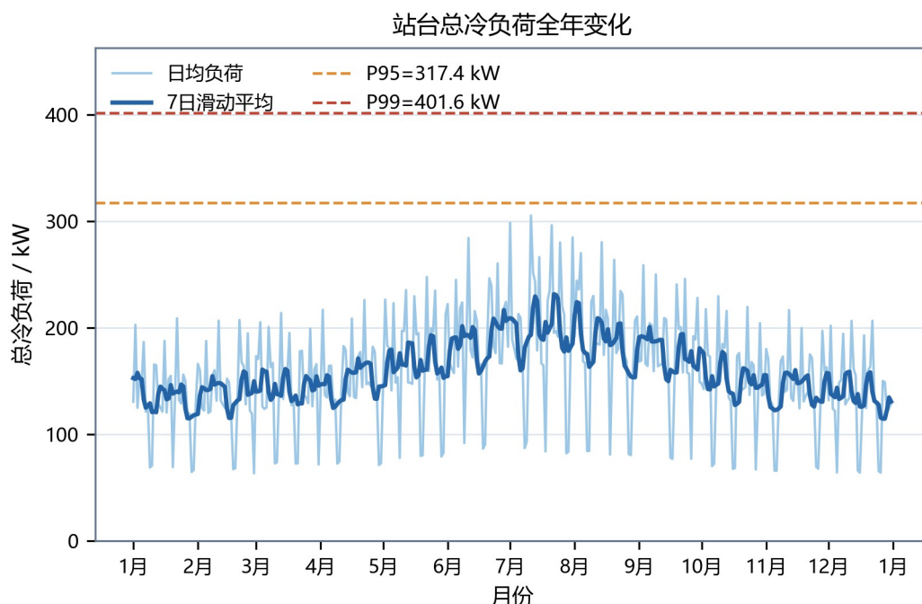
图 3-1 站台总冷负荷时间序列图
