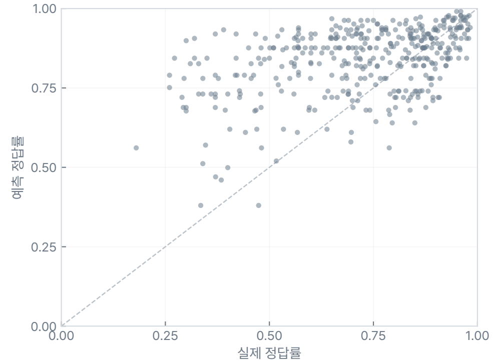
gpt-5.6-terra
