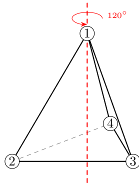
Rotation (234)
