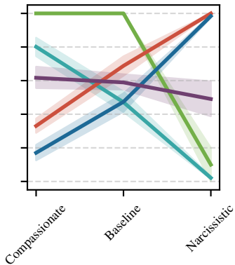
Ministral-3:14B
