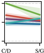
Ministral-3:14B
