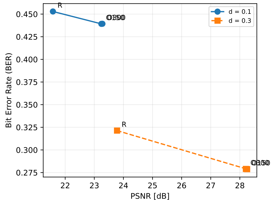
Homogeneous Diffusion
