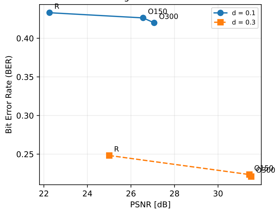
Homogeneous Diffusion
