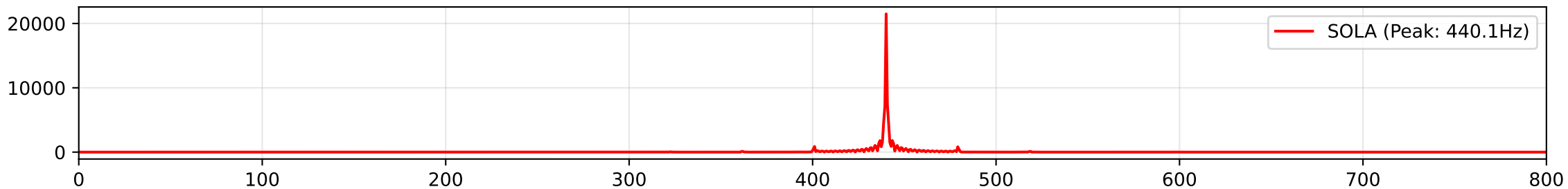
SOLA FFT (Stretch x1.41)
