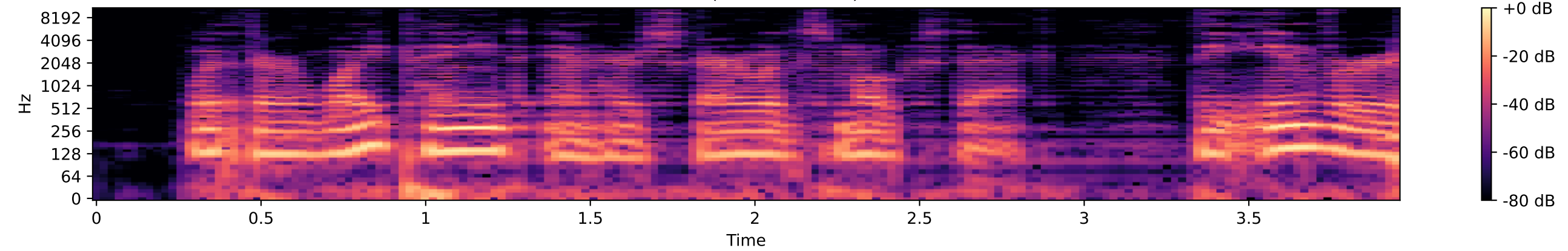
WSOLA (+6 semitones)
