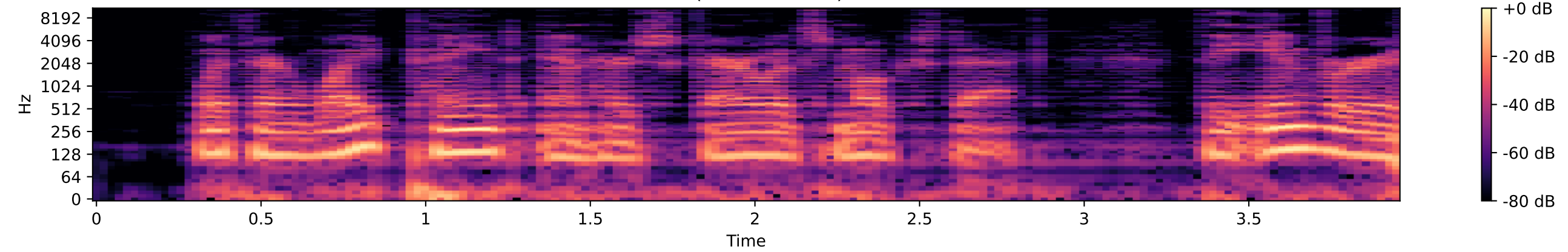
SOLA (+6 semitones)
