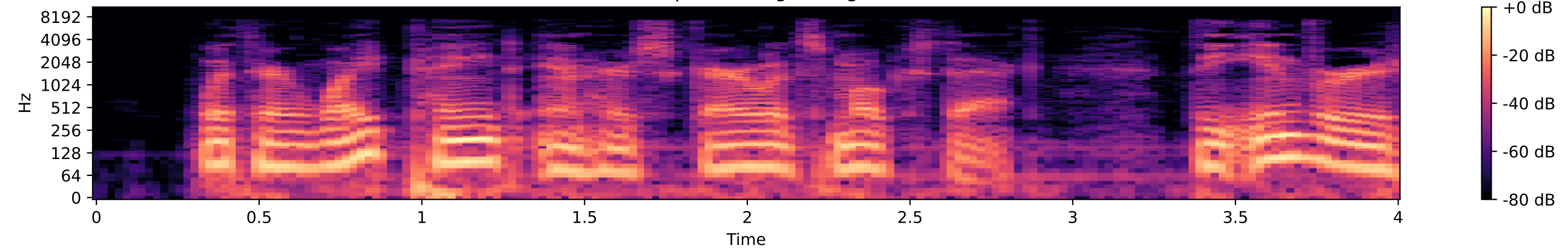
OLA (+6 semitones)
