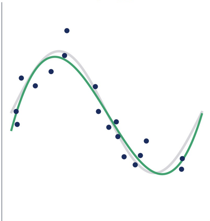
3차: 적절
