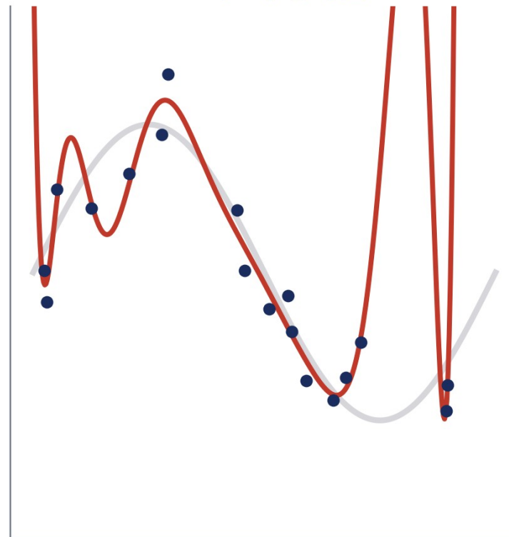
12차: 과대적합
