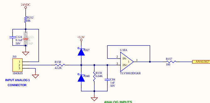
ANALOG INPUTS
