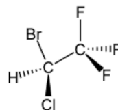
化合物 Q
