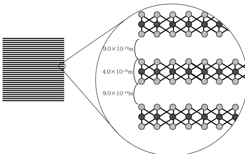
図 1-6 層状の \text{TaS}_2
