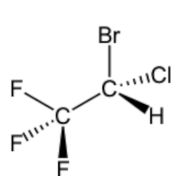
化合物 N
