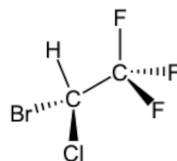
化合物 P
