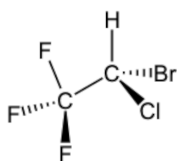
化合物 O
