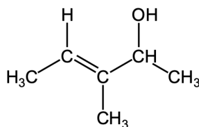
図 3-5 構造式の例
