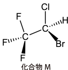
ハロタンの鏡像異性体のうちのひとつ
