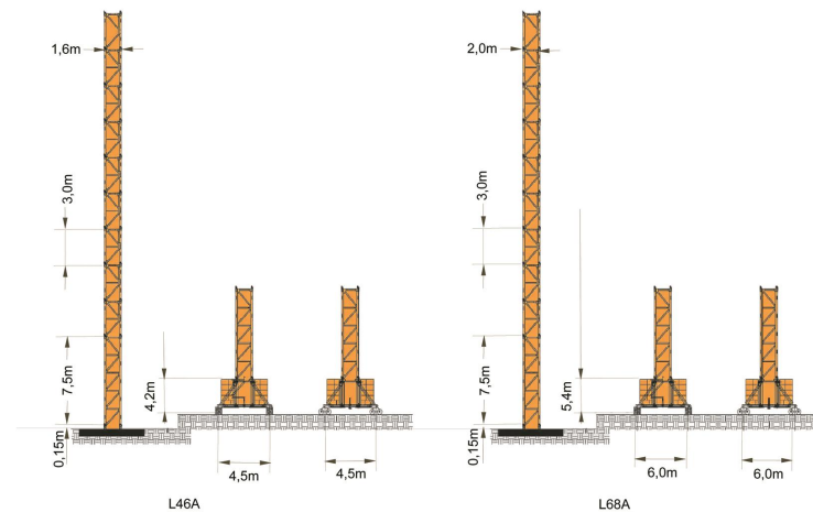
Tower configuration 塔身组成
