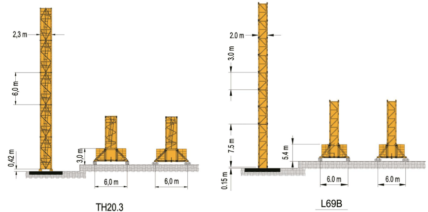
Tower configuration 塔身组成
