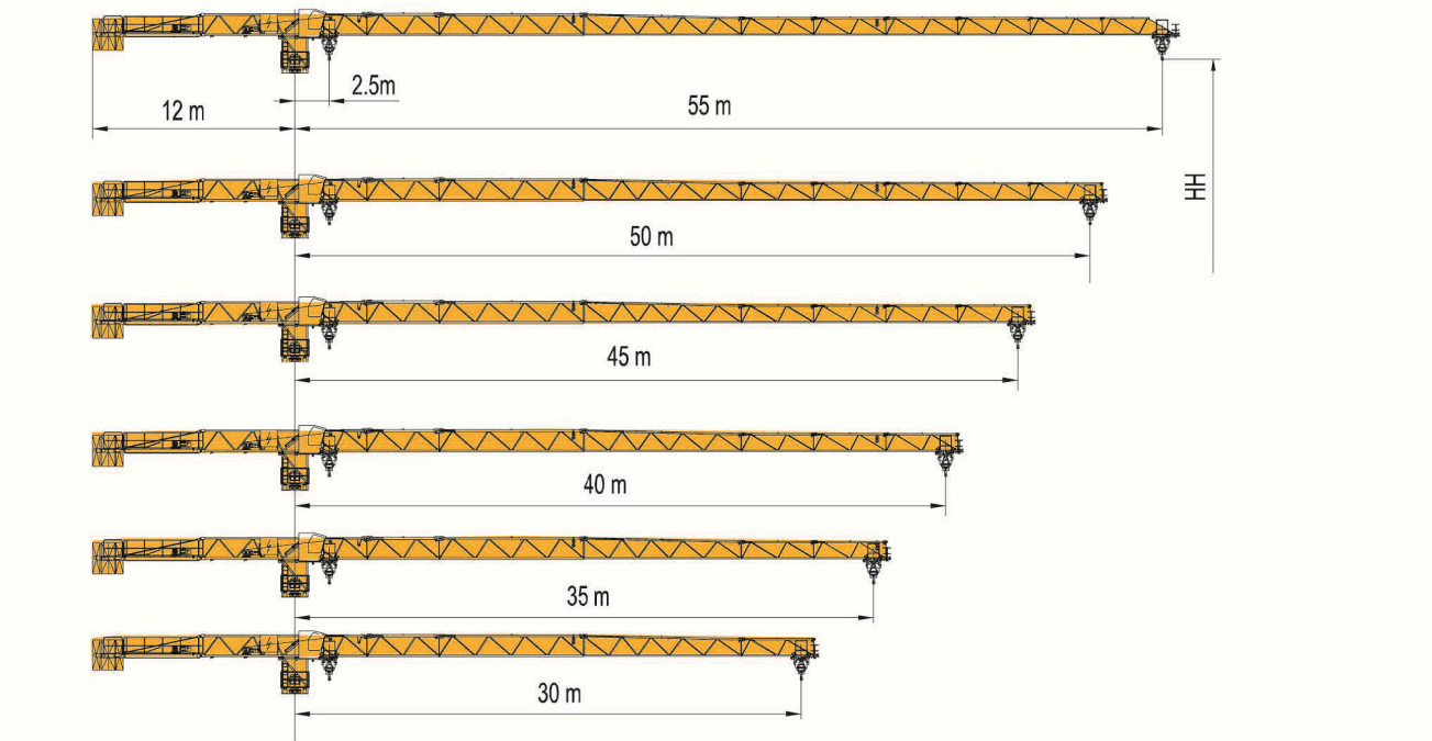
载荷特性 Load Diagrams
